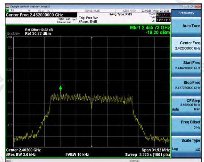
CH11
