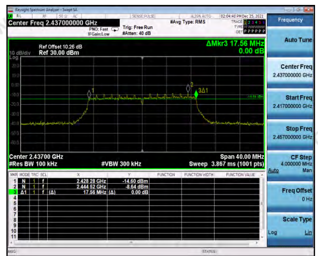
CH06
