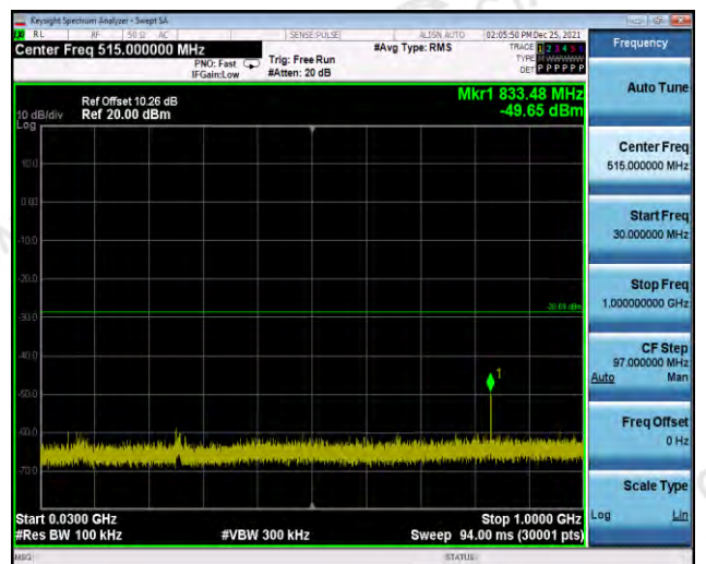
30MHz-3GHz
