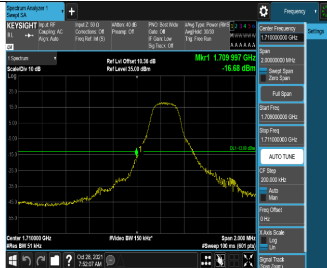
Band4-3MHz-QPSK-19965-1RB#14
