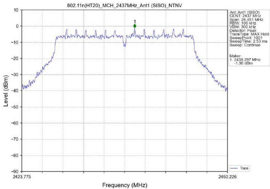
802.11n(HT20)_MCH_2437MHz_Ant1 (SISO)_NTNV
