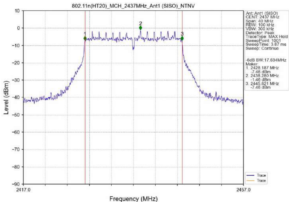
802.11n(HT20)_MCH_2437MHz_Ant1 (SISO)_NTNV
