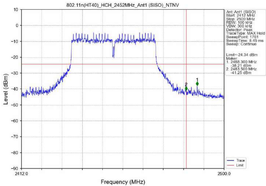
802.11n(HT40)_HCH_2452MHz_Ant1 (SISO)_NTNV
