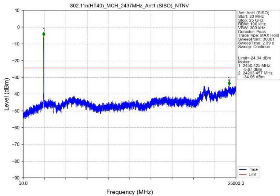
802.11n(HT40)_MCH_2437MHz_Ant1 (SISO)_NTNV
