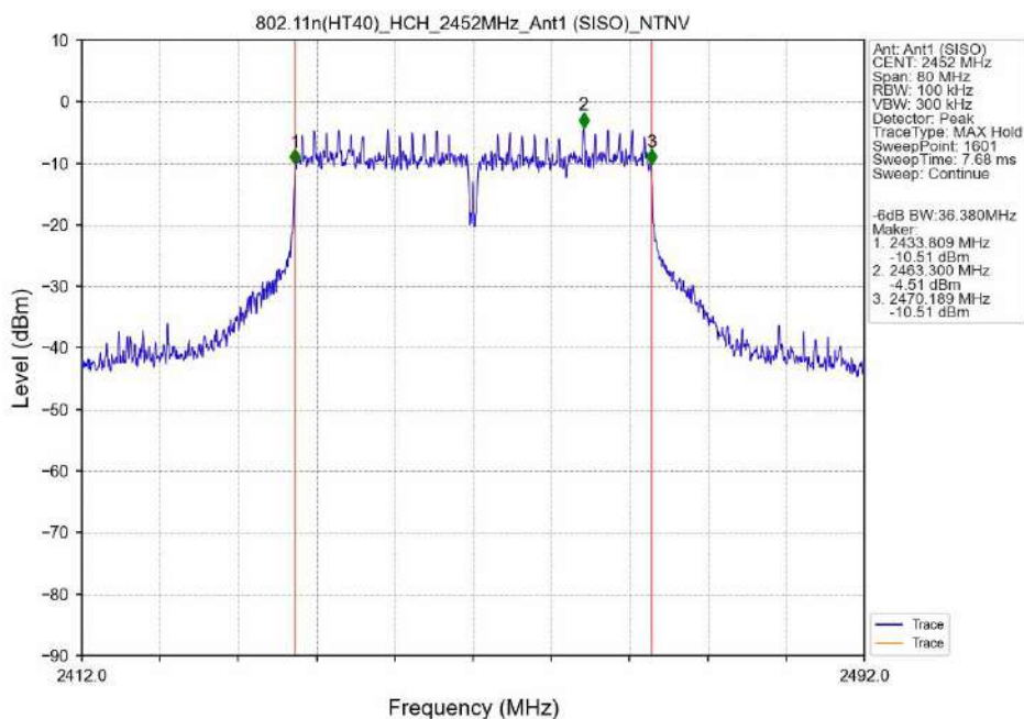
802.11n(HT40)_HCH_2452MHz_Ant1 (SISO)_NTNV
