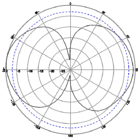
E (460MHz)
