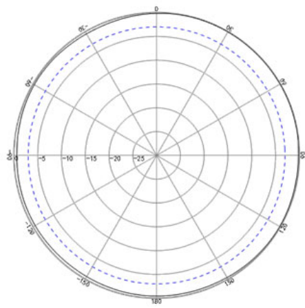
H (460MHz)
