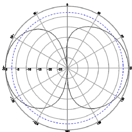
E (470MHz)
