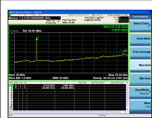
802.11ac(HT40)
