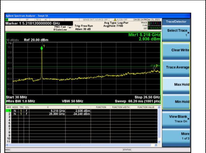
802.11ac(HT40)
