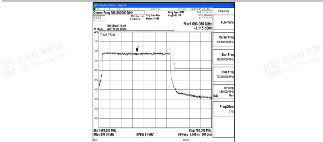
Band71_10MHz_QPSK_133422_50RB#0
