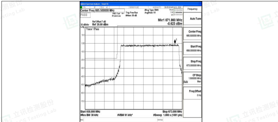
Band71_10MHz_QPSK_133172_50RB#0
