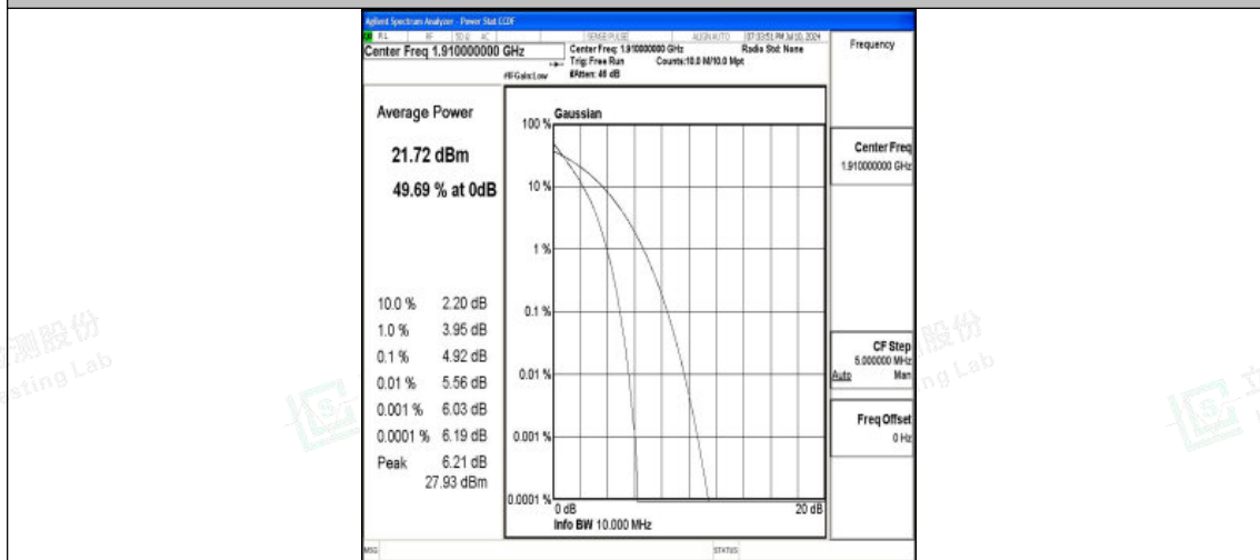
Band25-10MHz-QPSK-26640-50RB#0-PASS
