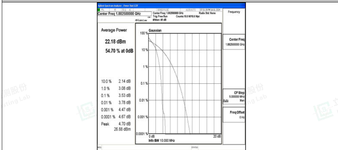
Band25-10MHz-QPSK-26365-1RB#0-PASS
