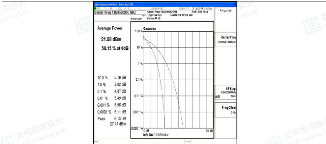
Band25-10MHz-QPSK-26365-50RB#0-PASS
