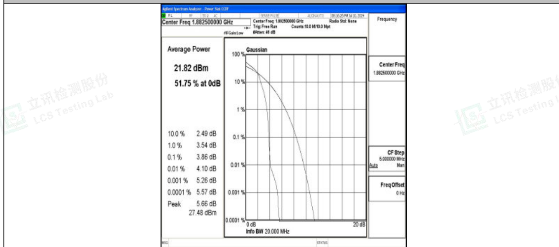
Band25-20MHz-16QAM-26365-1RB#0-PASS
