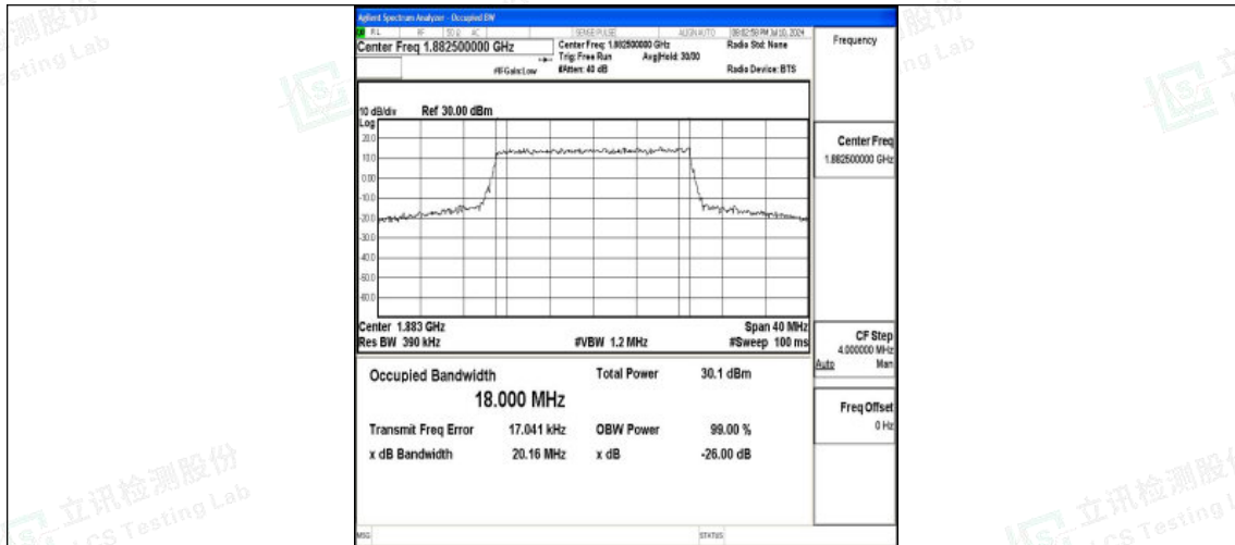
Band25-20MHz-16QAM-26365-100RB#0-PASS
