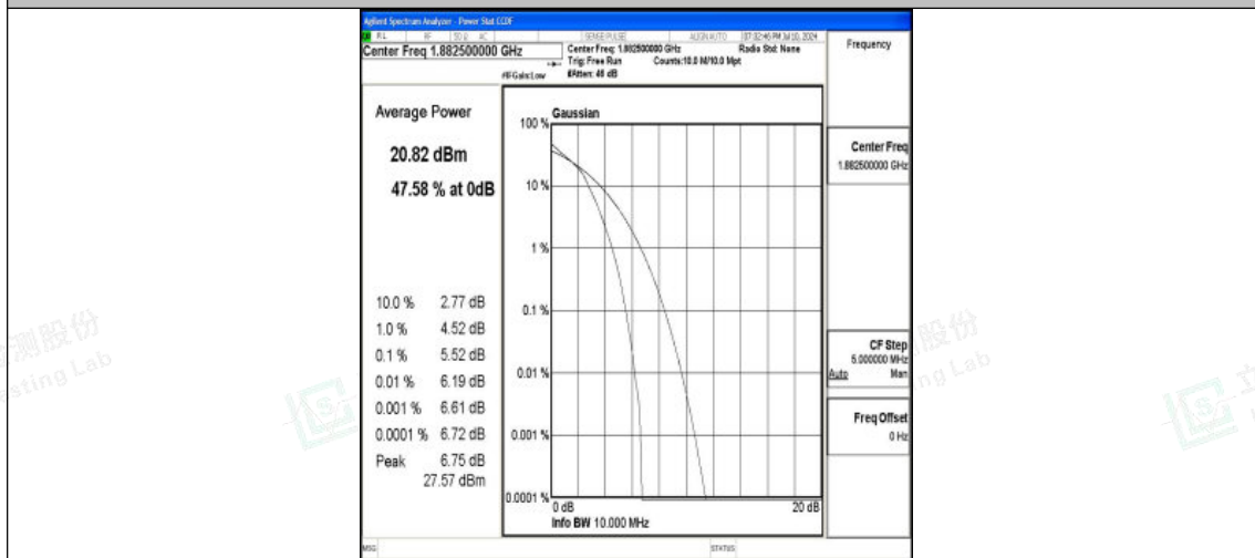
Band25-10MHz-16QAM-26365-50RB#0-PASS
