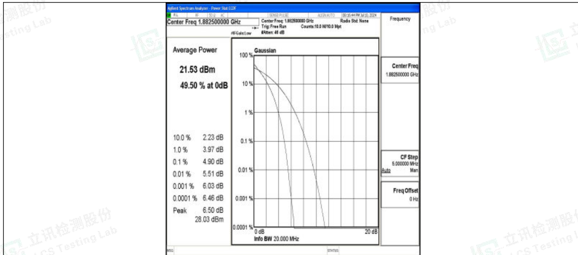
Band25-20MHz-QPSK-26365-100RB#0-PASS
