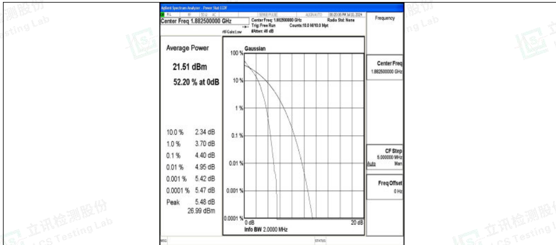
Band25-1.4MHz-QPSK-26365-6RB#0-PASS
