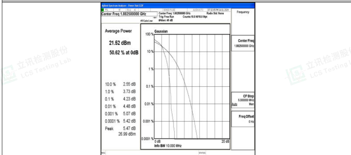
Band25-10MHz-16QAM-26365-1RB#0-PASS
