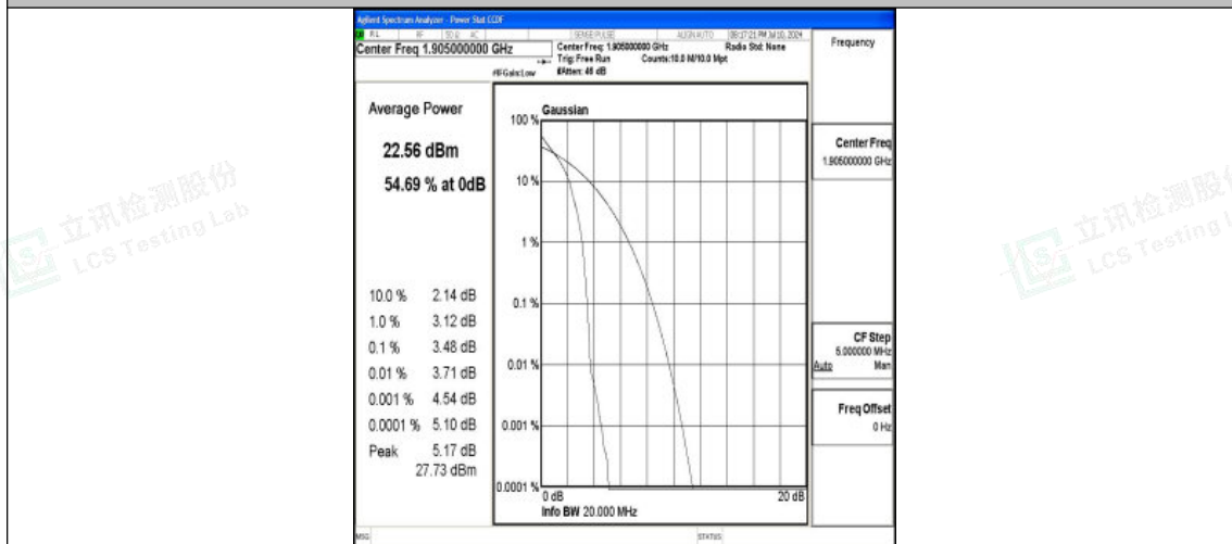
Band25-20MHz-QPSK-26590-1RB#0-PASS
