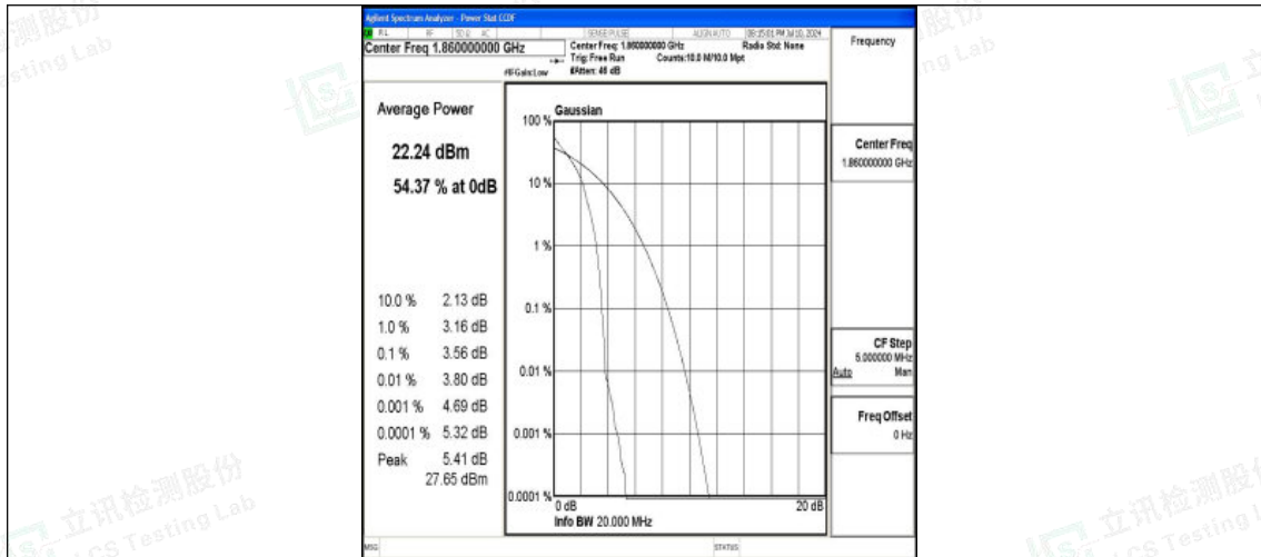
Band25-20MHz-QPSK-26140-1RB#0-PASS
