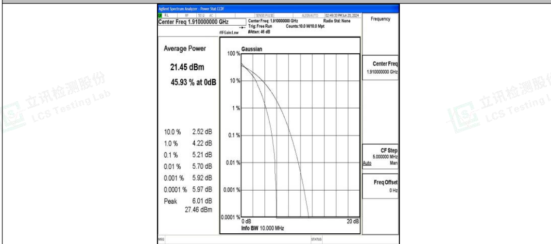
Band25-10MHz-QPSK-26640-1RB#0-PASS
