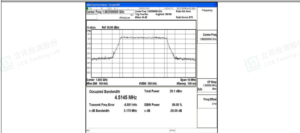
Band25-5MHz-QPSK-26365-25RB#0-PASS
