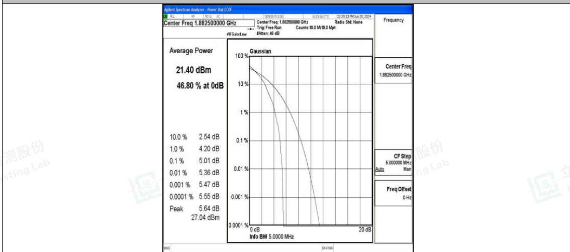
Band25-5MHz-QPSK-26365-1RB#0-PASS
