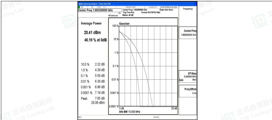
Band25-10MHz-QPSK-26365-50RB#0-PASS
