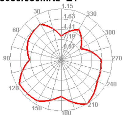
5650.000MHz E1
