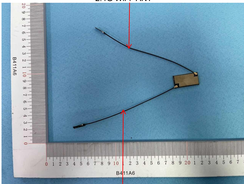
BLE-ANT
