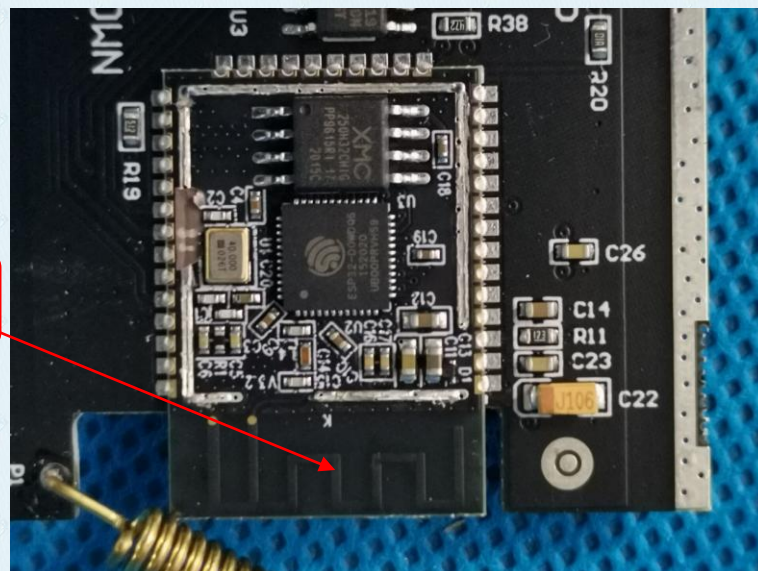
BT/WIFI Antenna
