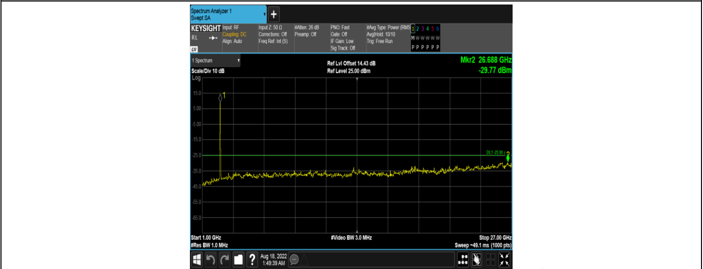
Band41-20MHz-16QAM-39750-1RB#0-Range2:1000~27000MHz
