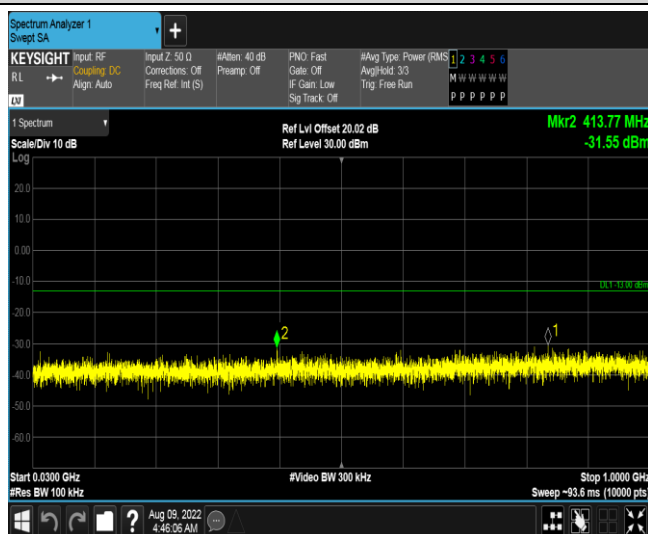
Band19-5MHz-QPSK-24125-1RB#0-Range1:30~1000MHz
