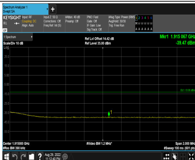
Band25-20MHz-QPSK-26590-1RB#99
