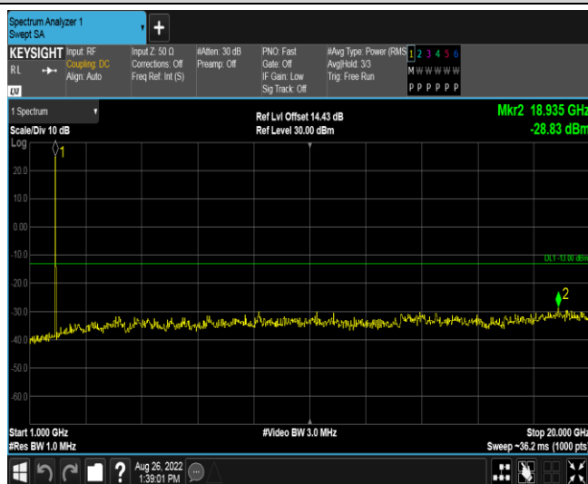
Band25-10MHz-QPSK-26365-1RB#0-Range2:1000~20000MHz
