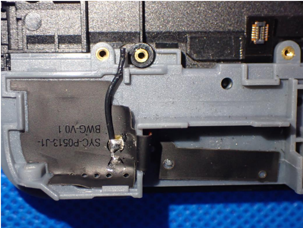
BT&WIFI&GPS ANTENNA
