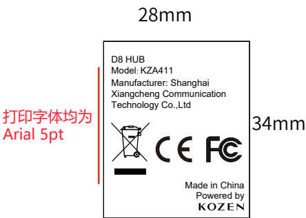
A0215机身标
