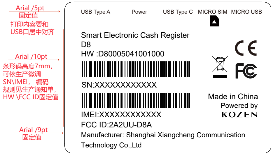
D0861机身标
