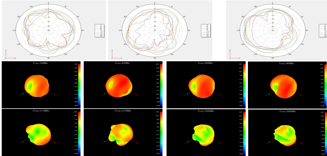
四、Antenna pattern
