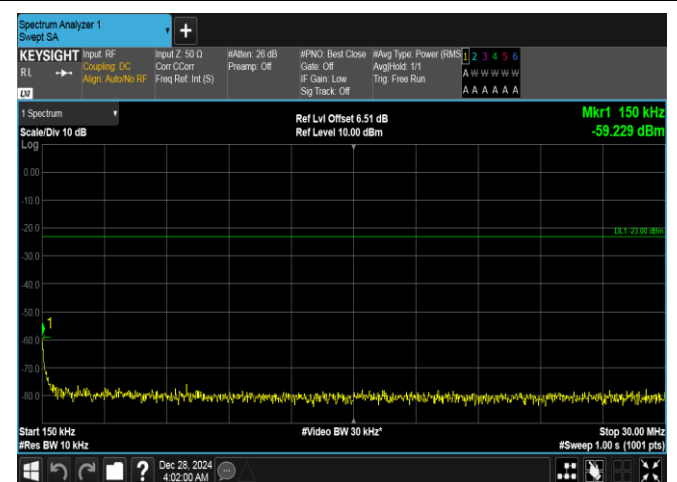
Band26(824-849)-10MHz-QPSK-26990-50RB#0-0.15~30-PASS
