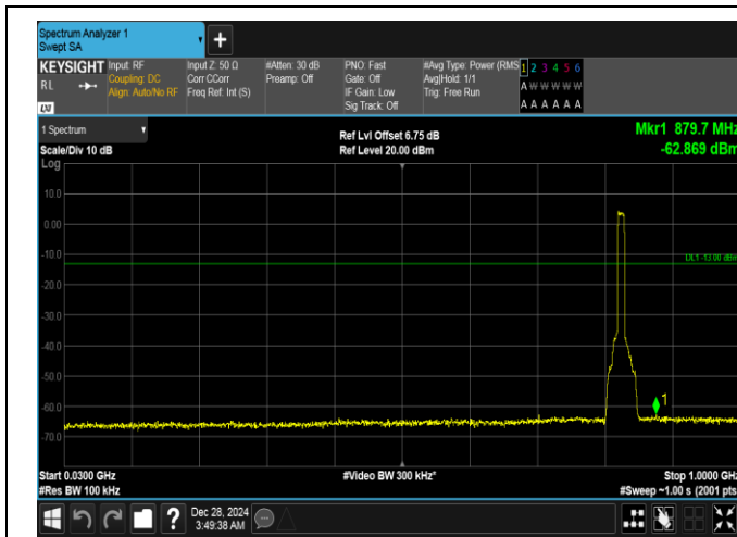
Band26(824-849)-10MHz-QPSK-26840-50RB#0-30~1000-PASS
