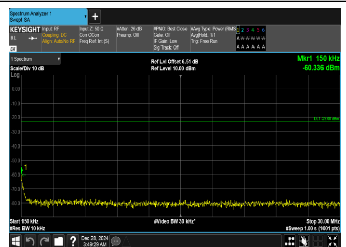
Band26(824-849)-10MHz-QPSK-26840-50RB#0-0.15~30-PASS
