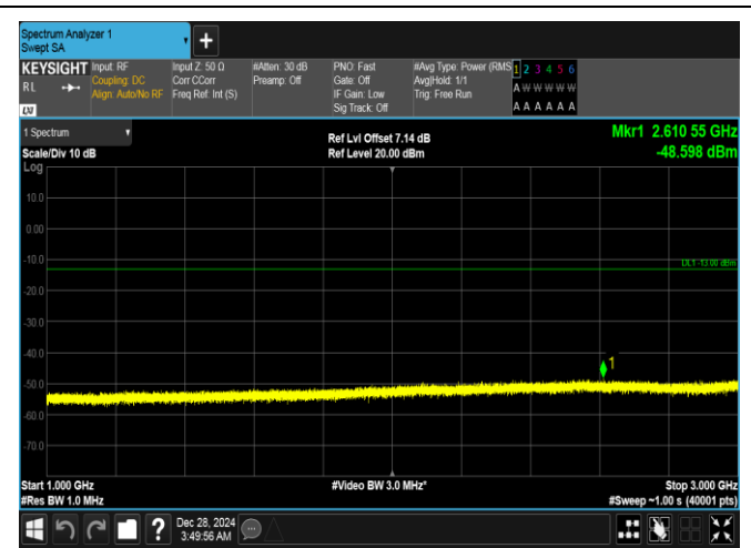
Band26(824-849)-10MHz-QPSK-26840-50RB#0-1000~3000-PASS
