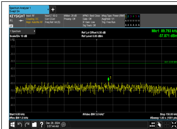
Band26(824-849)-10MHz-QPSK-26990-1RB#0-0.009~0.15-PASS
