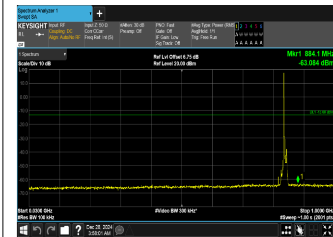
Band26(824-849)-10MHz-QPSK-26990-1RB#0-30~1000-PASS
