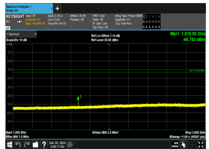
Band26(824-849)-10MHz-QPSK-26990-1RB#0-1000~3000-PASS
