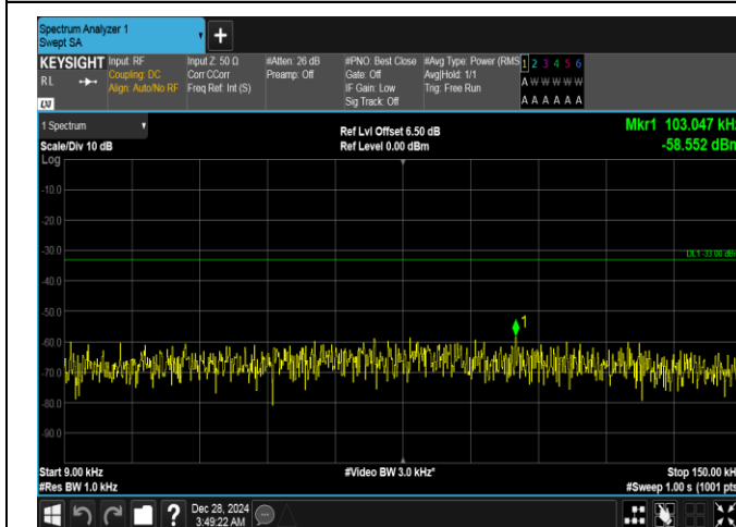
Band26(824-849)-10MHz-QPSK-26840-50RB#0-0.009~0.15-PASS
