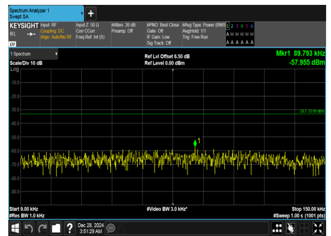
Band26(824-849)-10MHz-QPSK-26915-1RB#0-0.009~0.15-PASS
