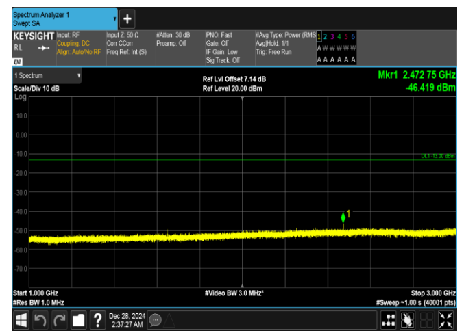
Band26(824-849)-3MHz-QPSK-26805-1RB#0-1000~3000-PASS
