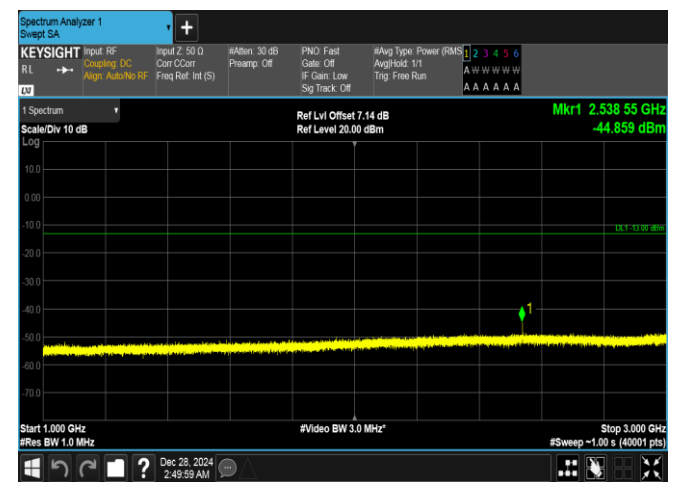
Band26(824-849)-3MHz-QPSK-27025-1RB#0-1000~3000-PASS
