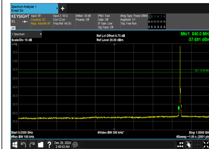
Band26(824-849)-3MHz-QPSK-27025-1RB#0-30~1000-PASS
