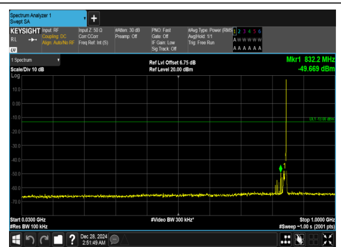
Band26(824-849)-3MHz-QPSK-27025-1RB#14-30~1000-PASS
