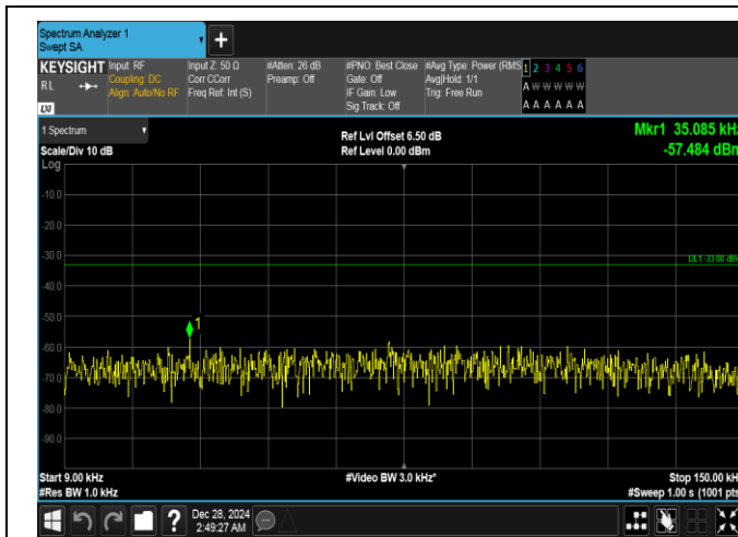
Band26(824-849)-3MHz-QPSK-27025-1RB#0-0.009~0.15-PASS
