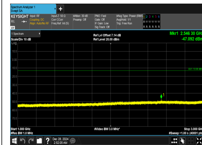
Band26(824-849)-3MHz-QPSK-27025-1RB#14-1000~3000-PASS
