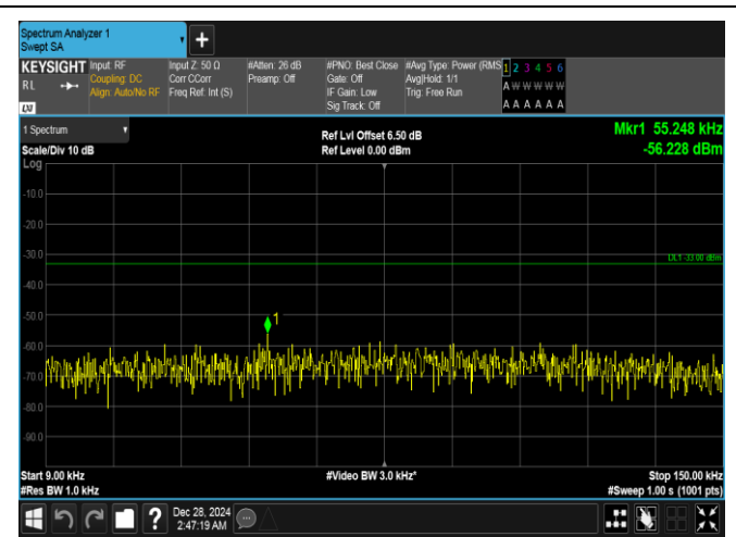
Band26(824-849)-3MHz-QPSK-26915-15RB#0-0.009~0.15-PASS
