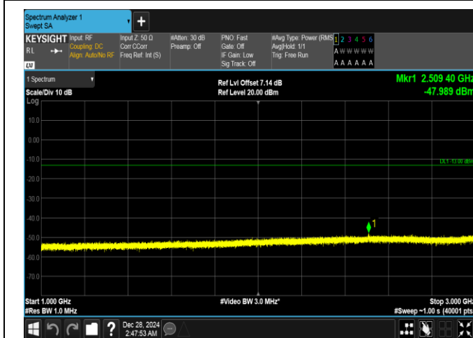
Band26(824-849)-3MHz-QPSK-26915-15RB#0-1000~3000-PASS
