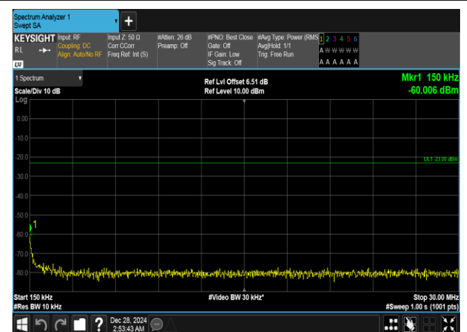
Band26(824-849)-3MHz-QPSK-27025-15RB#0-0.15~30-PASS
