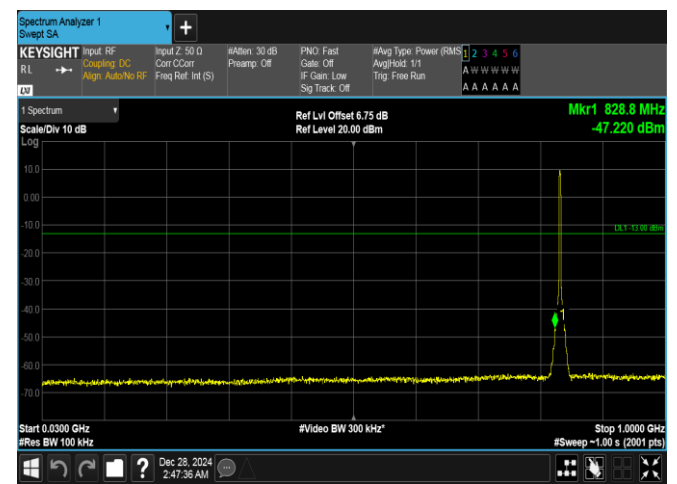
Band26(824-849)-3MHz-QPSK-26915-15RB#0-30~1000-PASS
