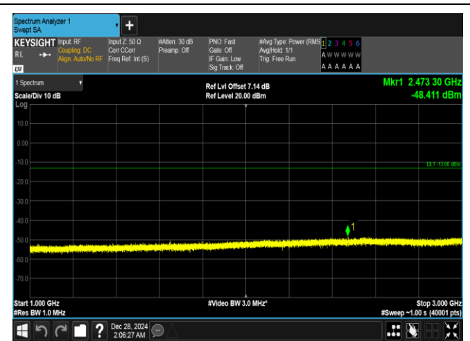
Band26(824-849)-1.4MHz-QPSK-26797-6RB#0-1000~3000-PASS
