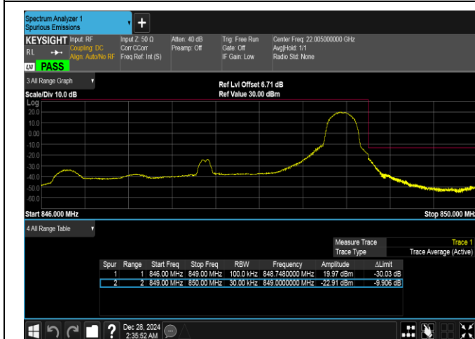
Band26(824-849)-3MHz-QPSK-27025-1RB#14-PASS
