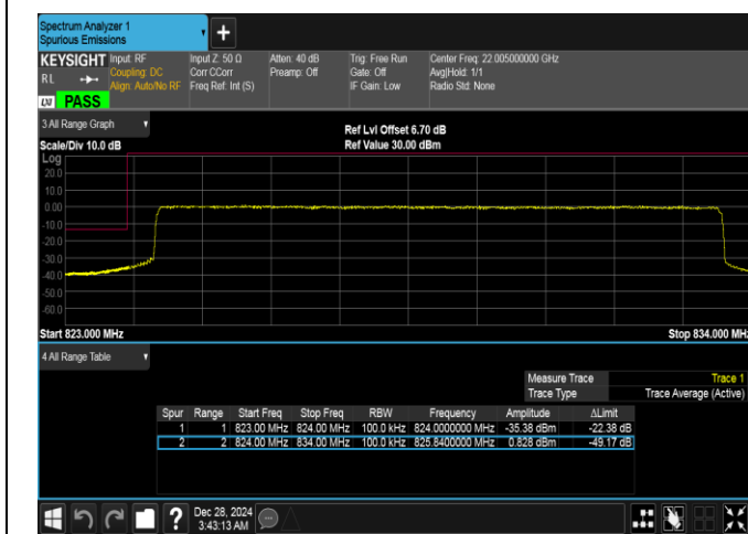
Band26(824-849)-10MHz-QPSK-26840-50RB#0-PASS
