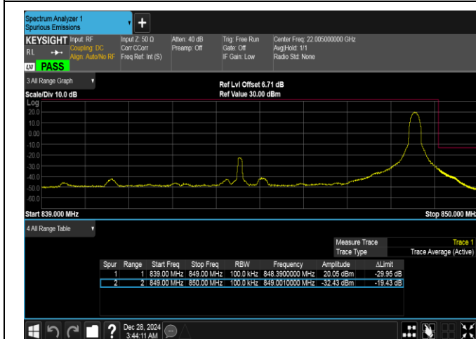
Band26(824-849)-10MHz-QPSK-26990-1RB#49-PASS
