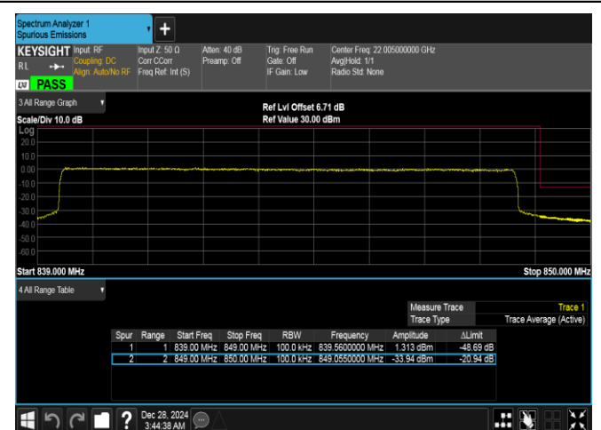
Band26(824-849)-10MHz-QPSK-26990-50RB#0-PASS
