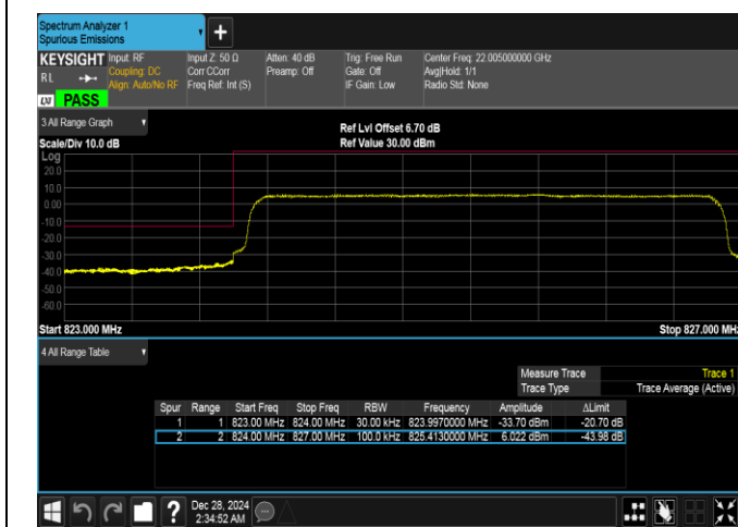
Band26(824-849)-3MHz-QPSK-26805-15RB#0-PASS
