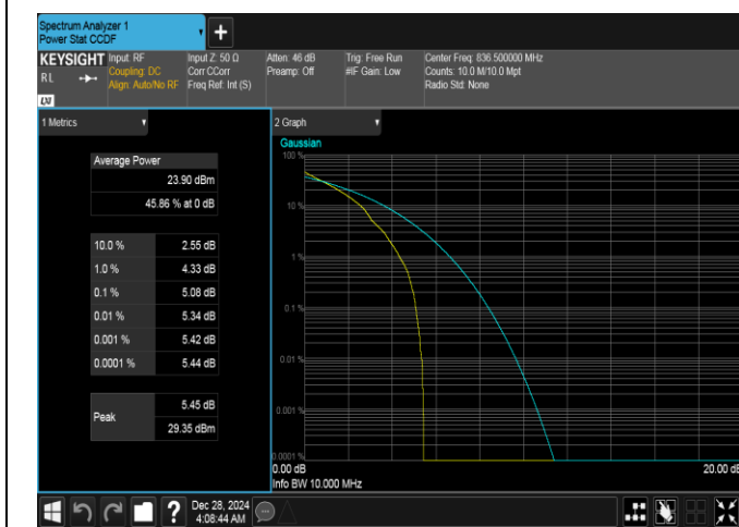
Band26(824-849)-10MHz-QPSK-26915-1RB#0-PASS
