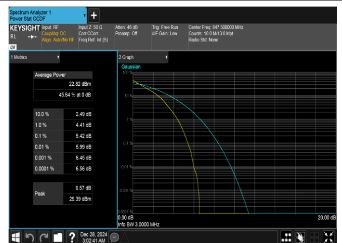
Band26(824-849)-3MHz-QPSK-27025-15RB#0-PASS
