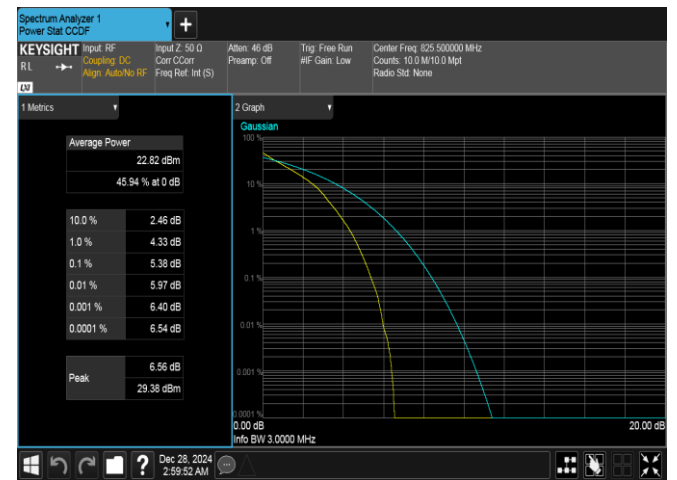
Band26(824-849)-3MHz-QPSK-26805-15RB#0-PASS
