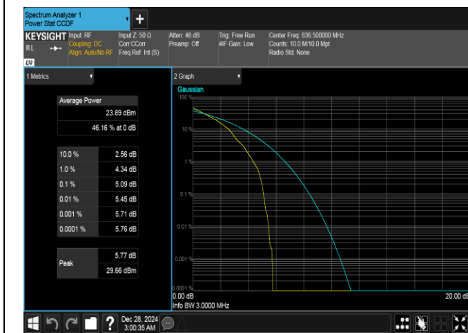
Band26(824-849)-3MHz-QPSK-26915-1RB#0-PASS
