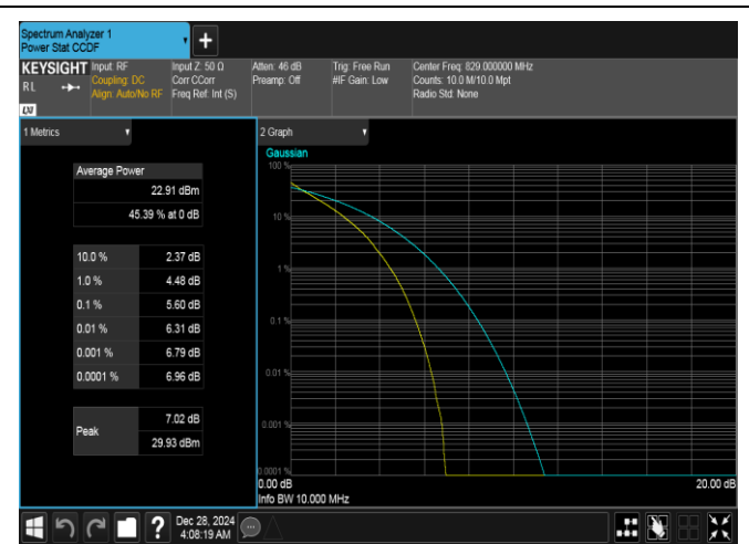
Band26(824-849)-10MHz-QPSK-26840-50RB#0-PASS
