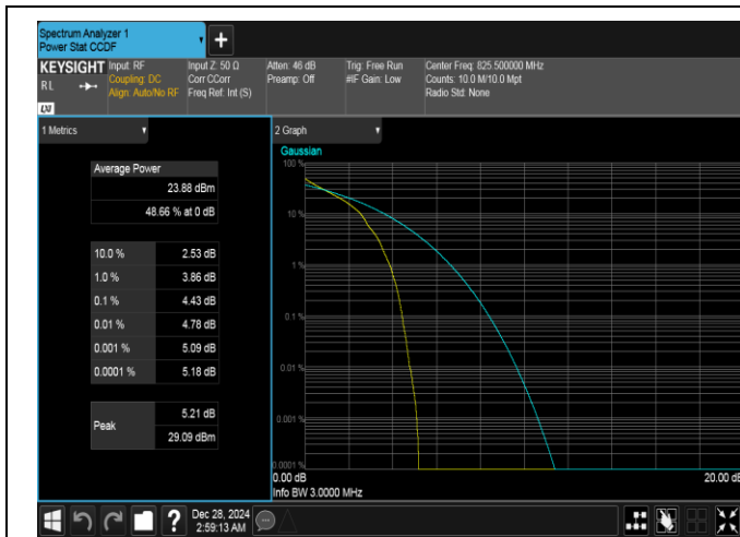
Band26(824-849)-3MHz-QPSK-26805-1RB#0-PASS
