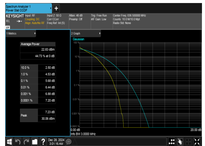
Band26(824-849)-3MHz-QPSK-26915-15RB#0-PASS
