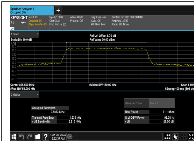
Band26(824-849)-3MHz-QPSK-26805-15RB#0-PASS
