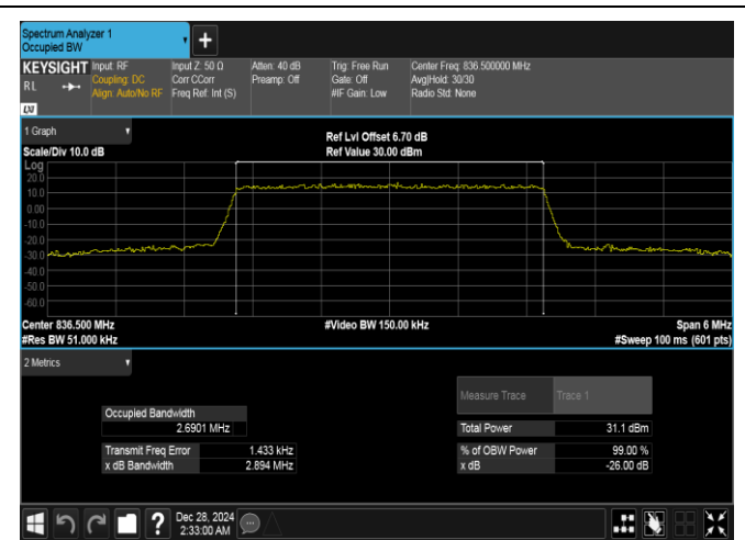
Band26(824-849)-3MHz-QPSK-26915-15RB#0-PASS
