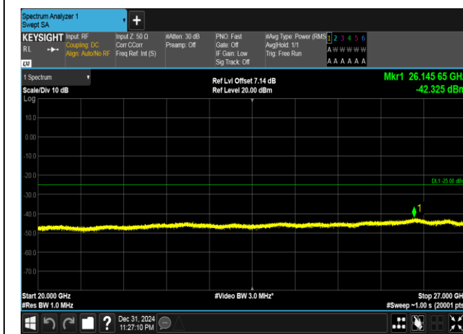
Band41(2535-2655)-20MHz-16QAM-40590-1RB#0-20000~27000-PASS
