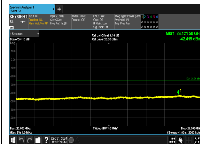
Band41(2535-2655)-20MHz-QPSK-40590-1RB#99-20000~27000-PASS
