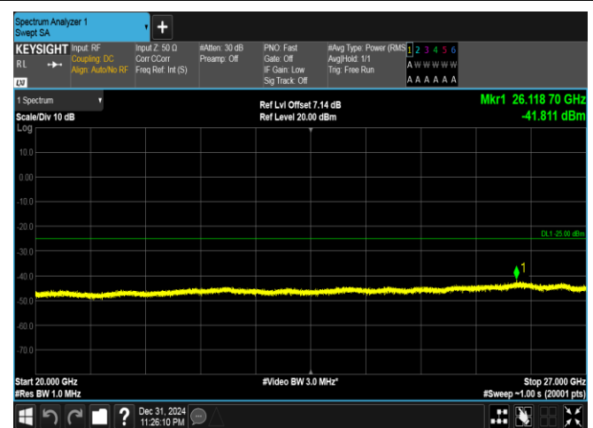
Band41(2535-2655)-20MHz-QPSK-40590-1RB#0-20000~27000-PASS
