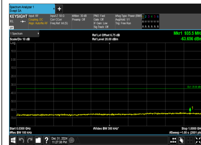
Band41(2535-2655)-20MHz-QPSK-40590-1RB#99-30~1000-PASS
