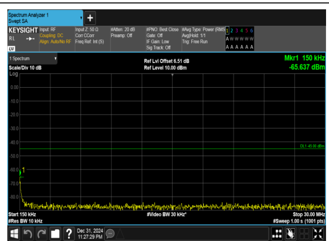
Band41(2535-2655)-20MHz-QPSK-40590-1RB#99-0.15~30-PASS
