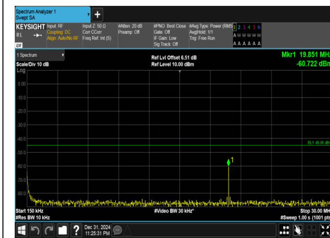
Band41(2535-2655)-20MHz-QPSK-40590-1RB#0-0.15~30-PASS
