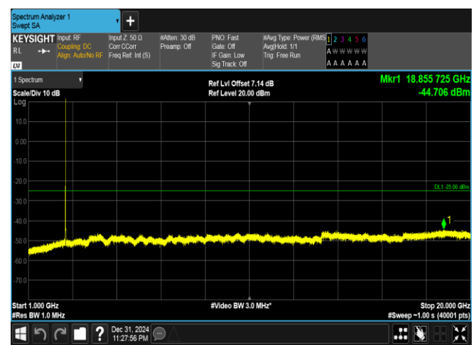
Band41(2535-2655)-20MHz-QPSK-40590-1RB#99-1000~20000-PASS
