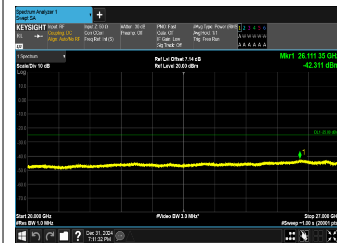
Band38-15MHz-QPSK-38175-1RB#0-20000~27000-PASS
