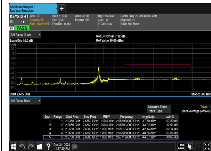
Band41(2535-2655)-20MHz-QPSK-41140-1RB#99-PASS
