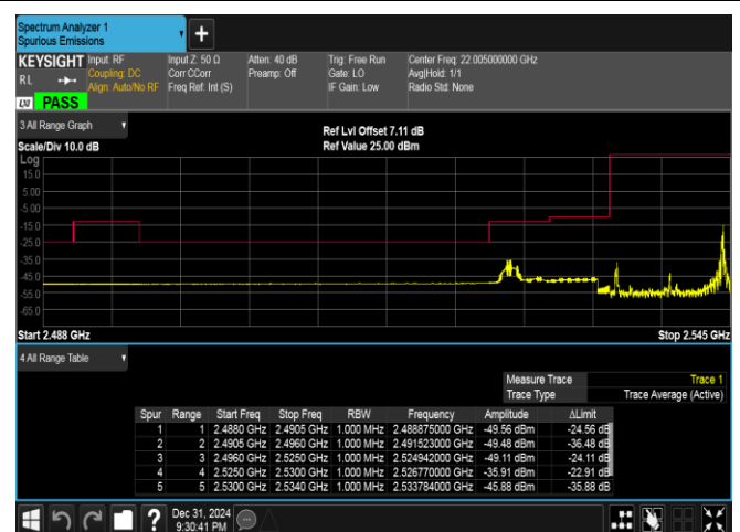
Band41(2535-2655)-10MHz-QPSK-40090-1RB#49-PASS
