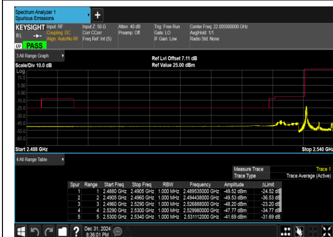
Band41(2535-2655)-5MHz-16QAM-40065-1RB#0-PASS
