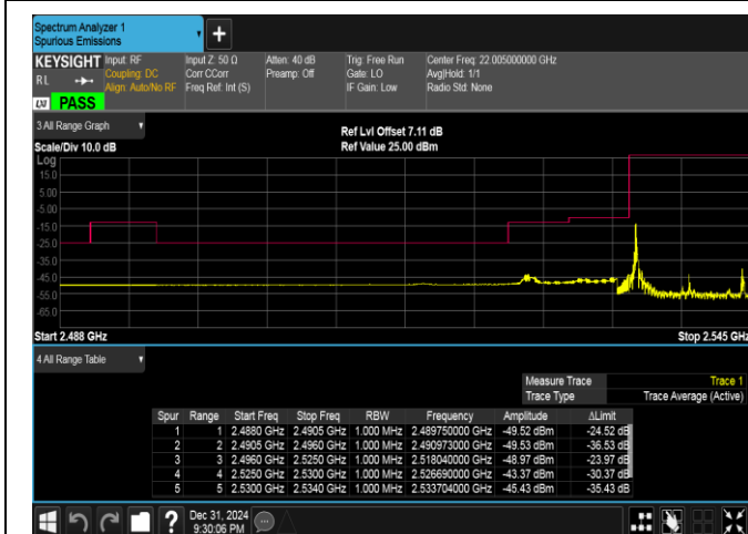
Band41(2535-2655)-10MHz-16QAM-40090-1RB#0-PASS
