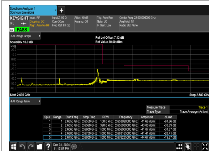
Band41(2535-2655)-20MHz-16QAM-41140-1RB#99-PASS
