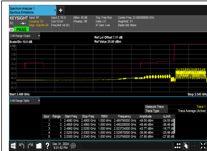
Band41(2535-2655)-10MHz-QPSK-40090-50RB#0-PASS
