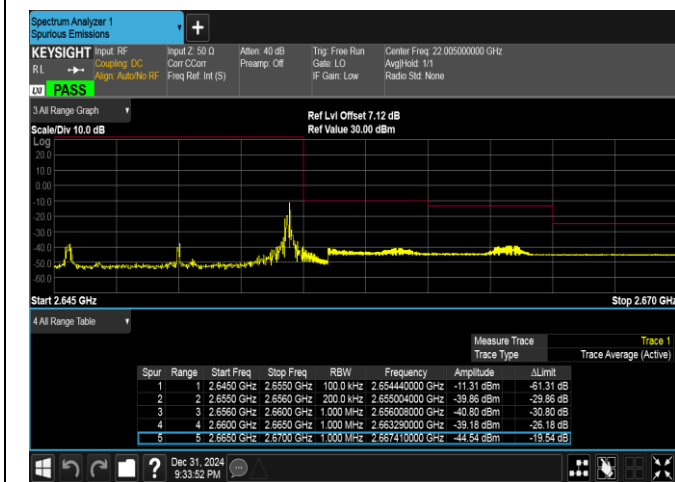
Band41(2535-2655)-10MHz-QPSK-41190-1RB#49-PASS
