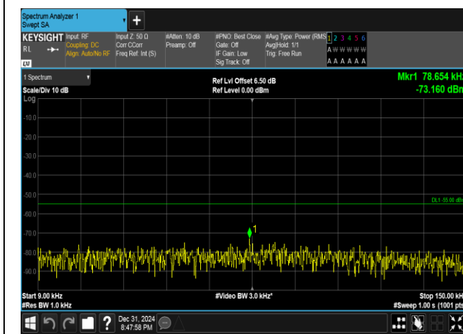
Band41(2535-2655)-5MHz-QPSK-40065-25RB#0-0.009~0.15-PASS
