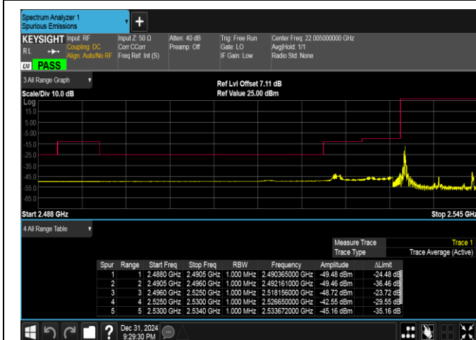
Band41(2535-2655)-10MHz-QPSK-40090-1RB#0-PASS
