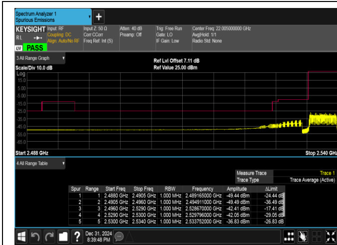
Band41(2535-2655)-5MHz-QPSK-40065-25RB#0-PASS
