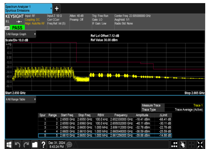
Band41(2535-2655)-5MHz-QPSK-41215-25RB#0-PASS
