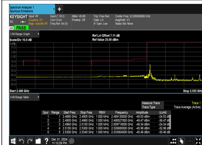
Band41(2535-2655)-20MHz-QPSK-40140-1RB#0-PASS
