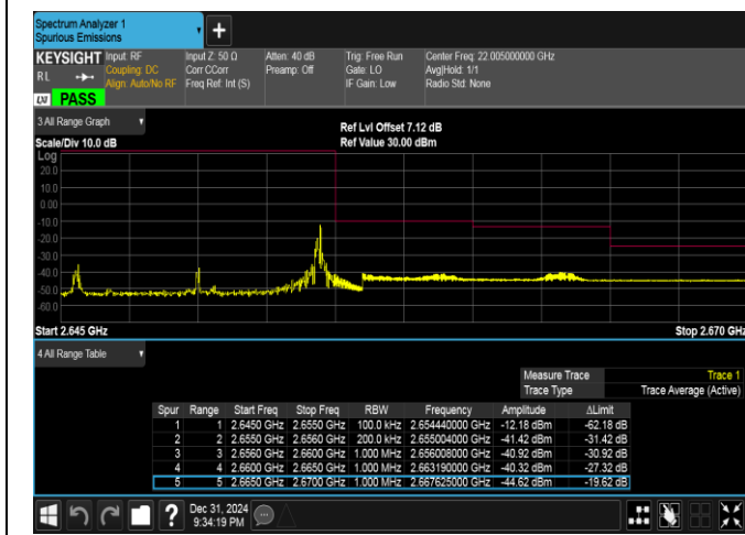
Band41(2535-2655)-10MHz-16QAM-41190-1RB#49-PASS
