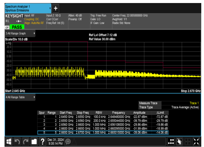
Band41(2535-2655)-10MHz-16QAM-41190-50RB#0-PASS
