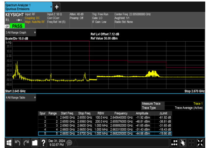
Band41(2535-2655)-10MHz-QPSK-41190-1RB#0-PASS
