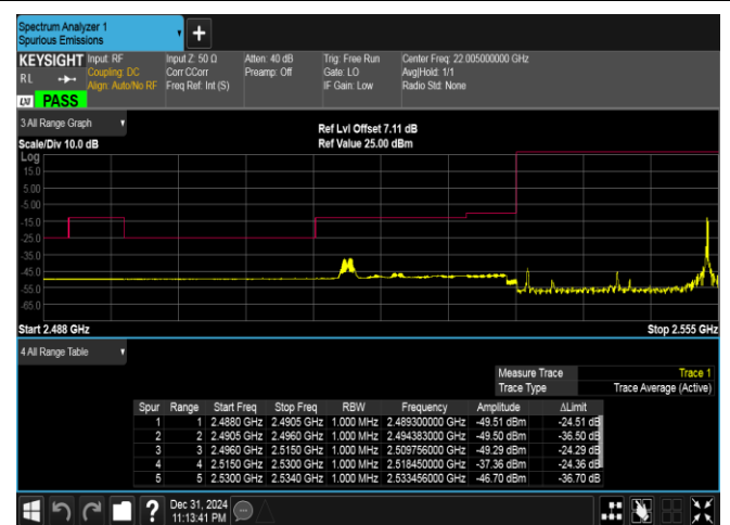
Band41(2535-2655)-20MHz-QPSK-40140-1RB#99-PASS
