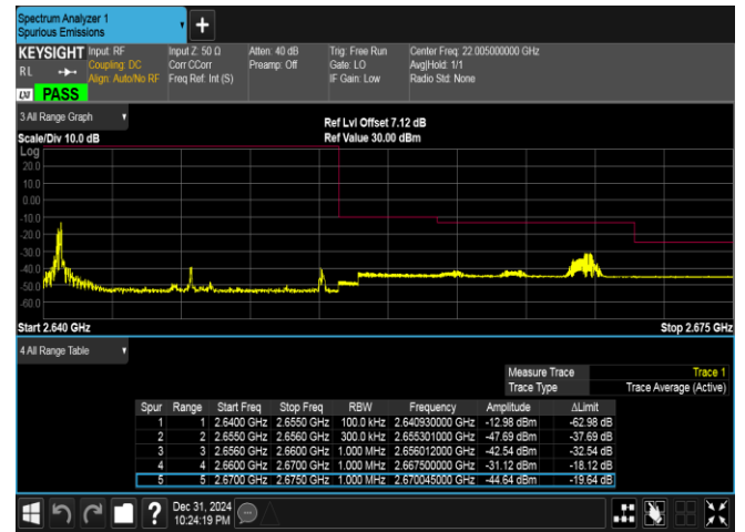
Band41(2535-2655)-15MHz-QPSK-41165-1RB#0-PASS
