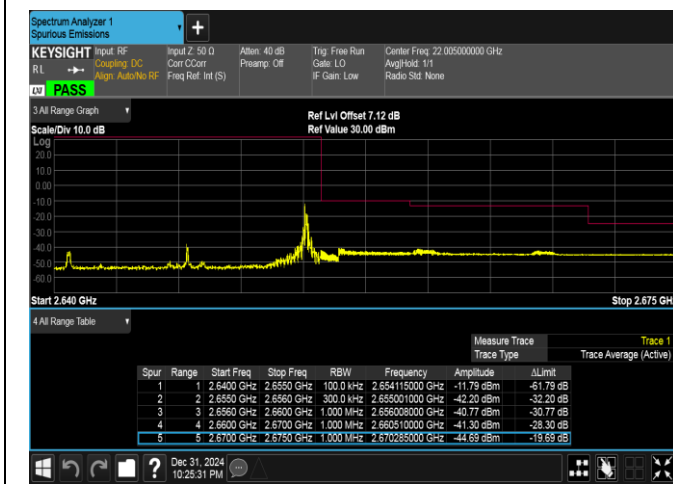
Band41(2535-2655)-15MHz-QPSK-41165-1RB#74-PASS
