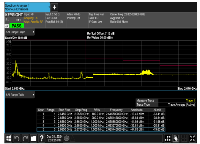
Band41(2535-2655)-10MHz-16QAM-41190-1RB#0-PASS
