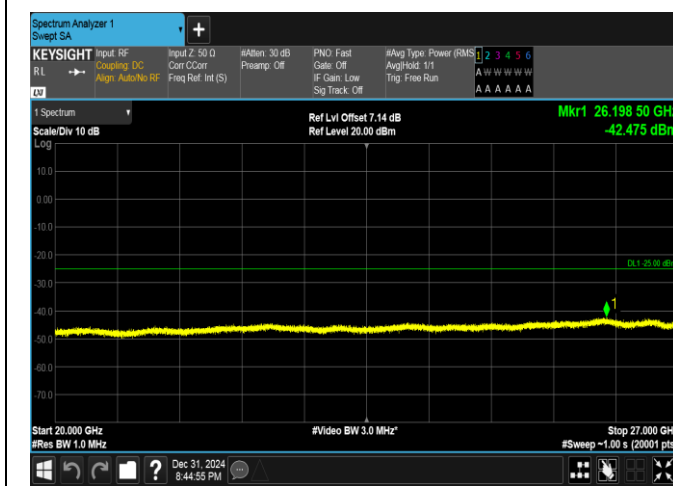
Band41(2535-2655)-5MHz-QPSK-40065-1RB#0-20000~27000-PASS
