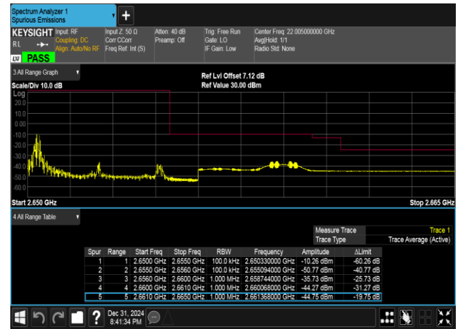
Band41(2535-2655)-5MHz-QPSK-41215-1RB#0-PASS
