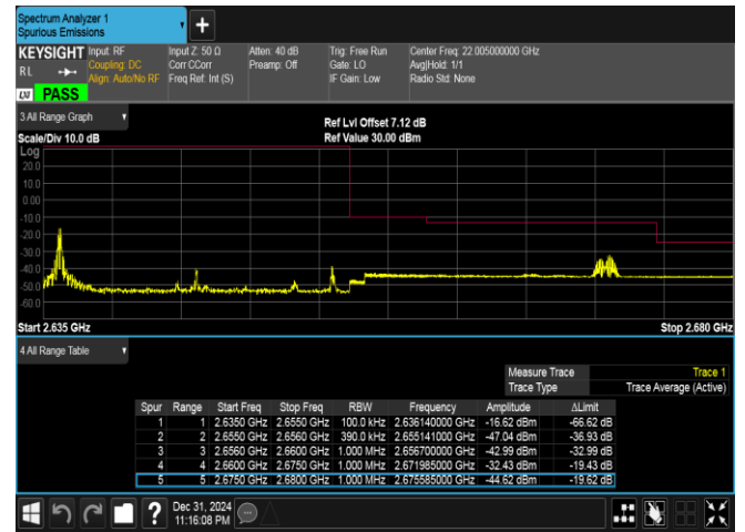
Band41(2535-2655)-20MHz-QPSK-41140-1RB#0-PASS
