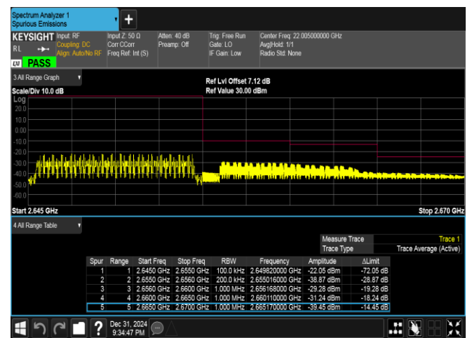
Band41(2535-2655)-10MHz-QPSK-41190-50RB#0-PASS
