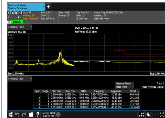
Band41(2535-2655)-5MHz-QPSK-41215-1RB#24-PASS
