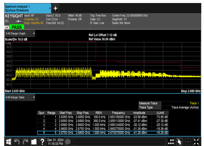
Band41(2535-2655)-20MHz-QPSK-41140-100RB#0-PASS
