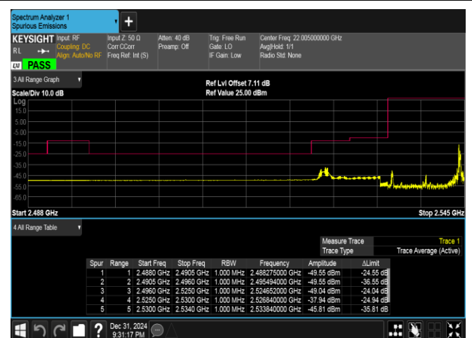
Band41(2535-2655)-10MHz-16QAM-40090-1RB#49-PASS
