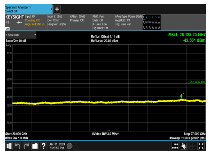
Band38-5MHz-QPSK-38000-25RB#0-20000~27000-PASS
