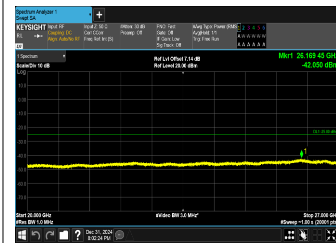
Band38-20MHz-QPSK-38150-1RB#0-20000~27000-PASS
