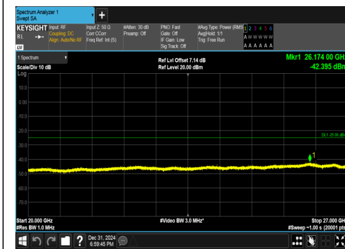
Band38-15MHz-QPSK-37825-1RB#0-20000~27000-PASS
