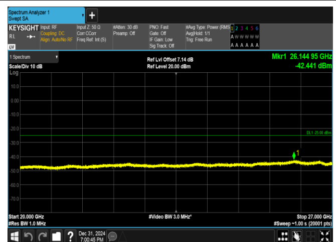
Band38-15MHz-16QAM-37825-1RB#0-20000~27000-PASS
