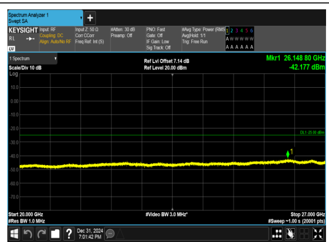
Band38-15MHz-QPSK-37825-1RB#74-20000~27000-PASS
