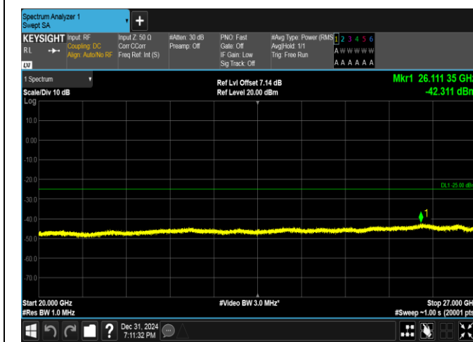
Band38-15MHz-QPSK-38175-1RB#0-20000~27000-PASS
