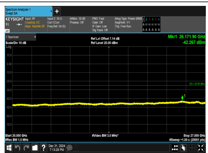
Band38-15MHz-QPSK-38175-1RB#74-20000~27000-PASS
