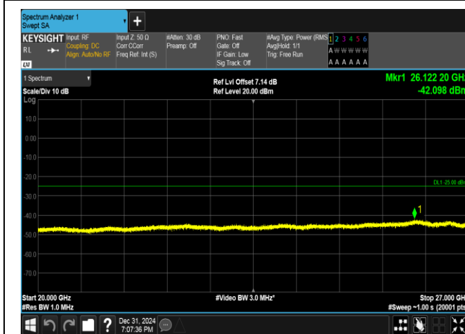
Band38-15MHz-QPSK-38000-1RB#74-20000~27000-PASS
