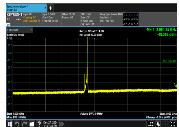
Band25-20MHz-16QAM-26590-1RB#99-1000~3000-PASS
