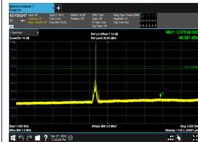
Band25-20MHz-QPSK-26140-1RB#99-1000~3000-PASS
