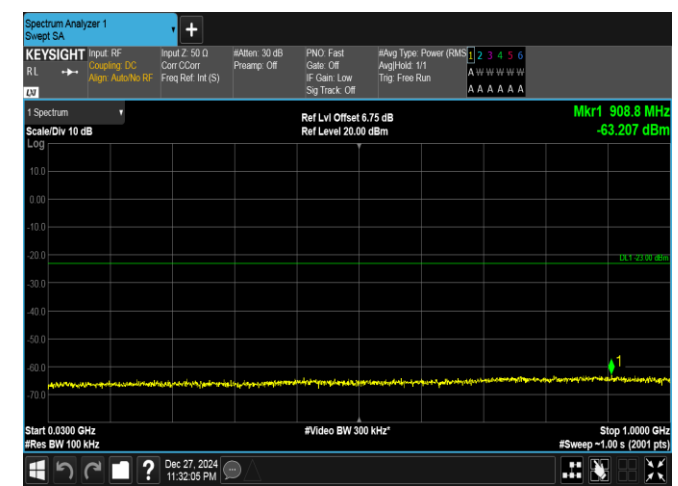
Band25-20MHz-QPSK-26365-100RB#0-30~1000-PASS
