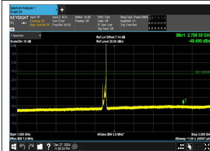
Band25-20MHz-QPSK-26590-1RB#99-1000~3000-PASS
