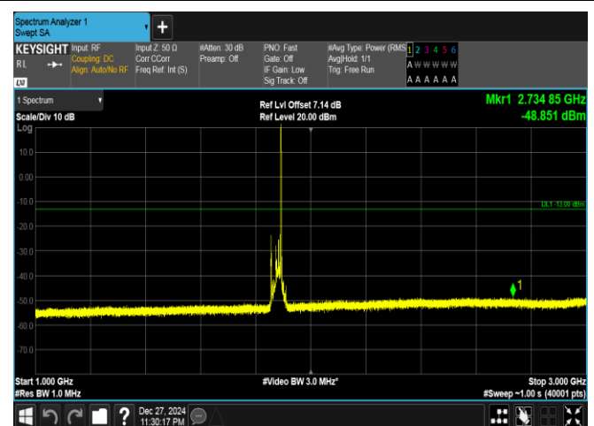
Band25-20MHz-QPSK-26365-1RB#99-1000~3000-PASS
