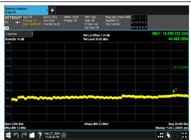
Band25-20MHz-QPSK-26365-1RB#0-3000~20000-PASS
