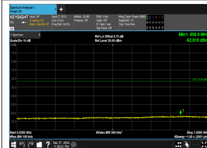
Band25-20MHz-QPSK-26365-1RB#99-30~1000-PASS
