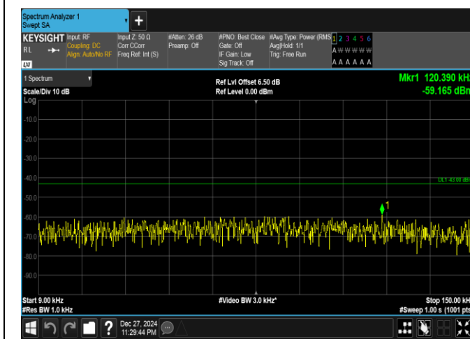
Band25-20MHz-QPSK-26365-1RB#99-0.009~0.15-PASS
