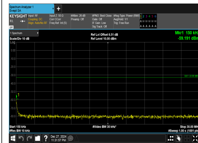
Band25-20MHz-QPSK-26365-100RB#0-0.15~30-PASS
