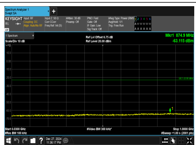
Band25-20MHz-QPSK-26590-1RB#99-30~1000-PASS
