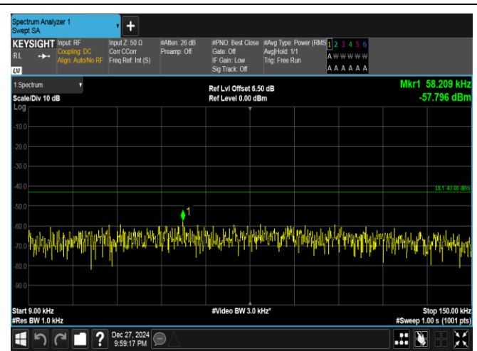
Band25-10MHz-QPSK-26365-50RB#0-0.009~0.15-PASS
