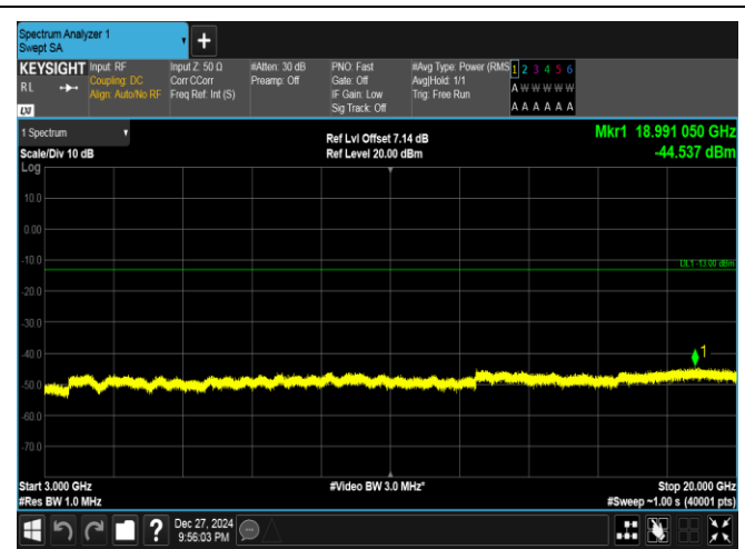
Band25-10MHz-QPSK-26365-1RB#0-3000~20000-PASS
