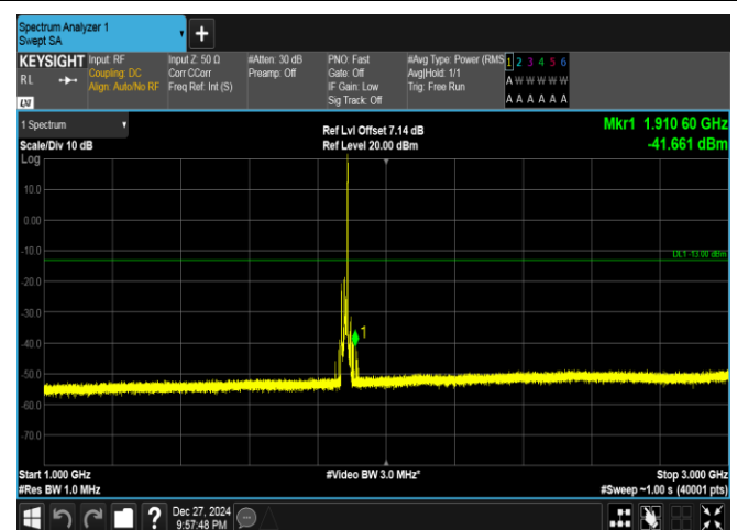
Band25-10MHz-QPSK-26365-1RB#49-1000~3000-PASS
