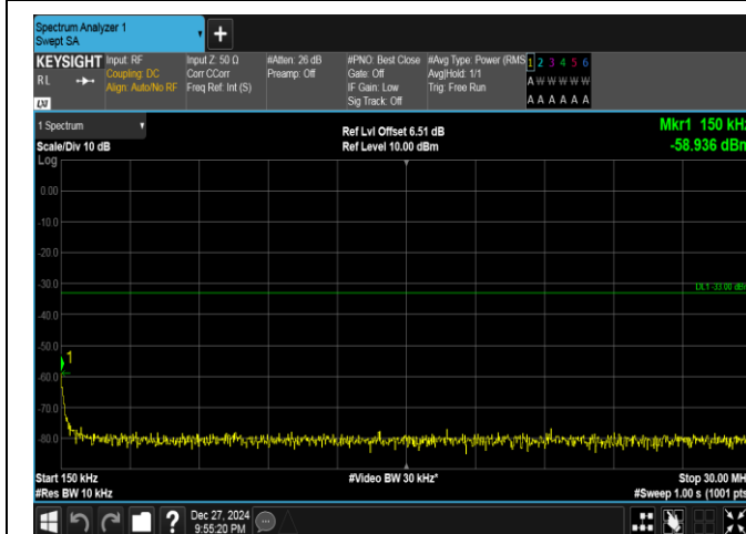
Band25-10MHz-QPSK-26365-1RB#0-0.15~30-PASS
