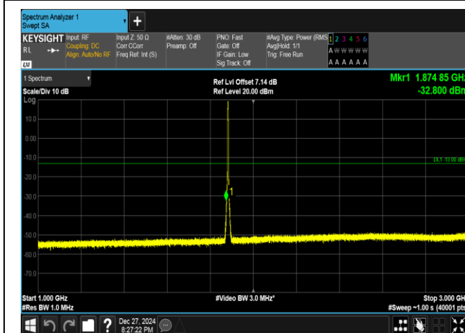
Band25-3MHz-QPSK-26365-15RB#0-1000~3000-PASS
