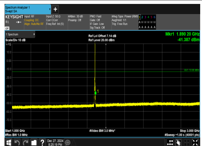
Band25-3MHz-QPSK-26365-1RB#14-1000~3000-PASS
