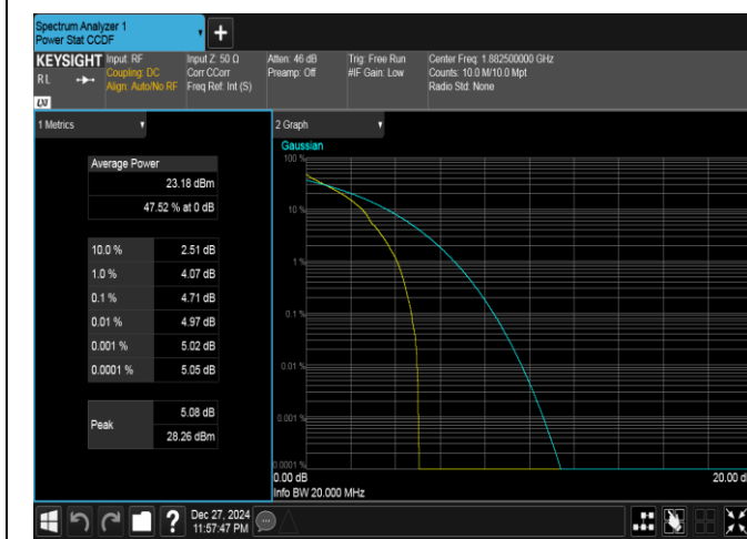
Band25-20MHz-QPSK-26365-1RB#0-PASS
