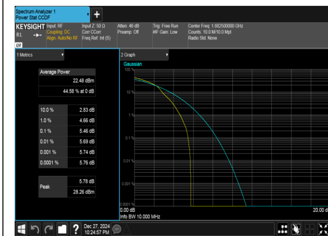
Band25-10MHz-16QAM-26365-1RB#0-PASS
