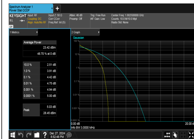
Band25-3MHz-QPSK-26365-1RB#0-PASS
