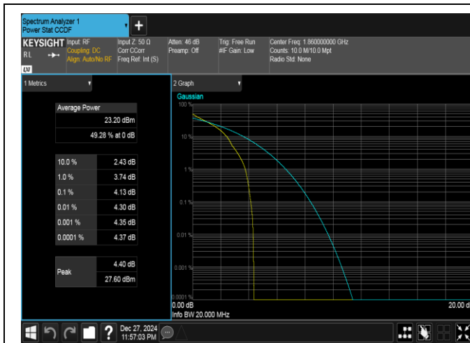
Band25-20MHz-QPSK-26140-1RB#0-PASS
