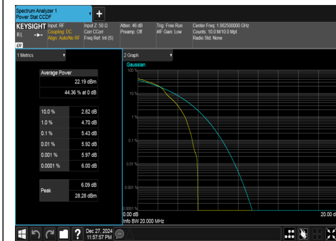
Band25-20MHz-16QAM-26365-1RB#0-PASS
