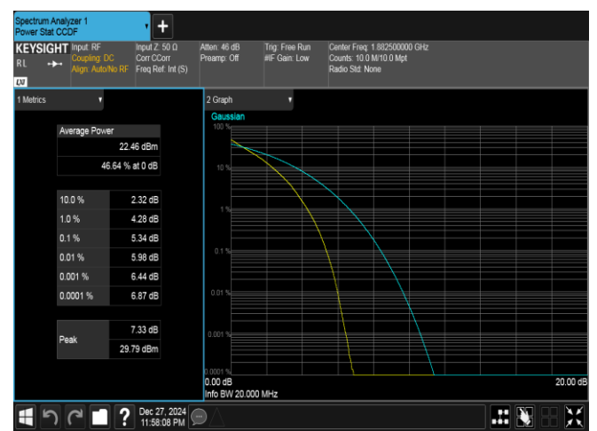
Band25-20MHz-QPSK-26365-100RB#0-PASS
