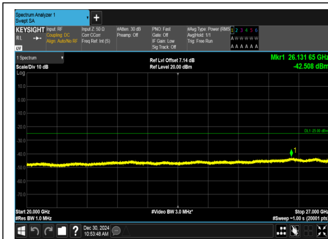
Band7-20MHz-QPSK-20850-100RB#0-20000~27000-PASS
