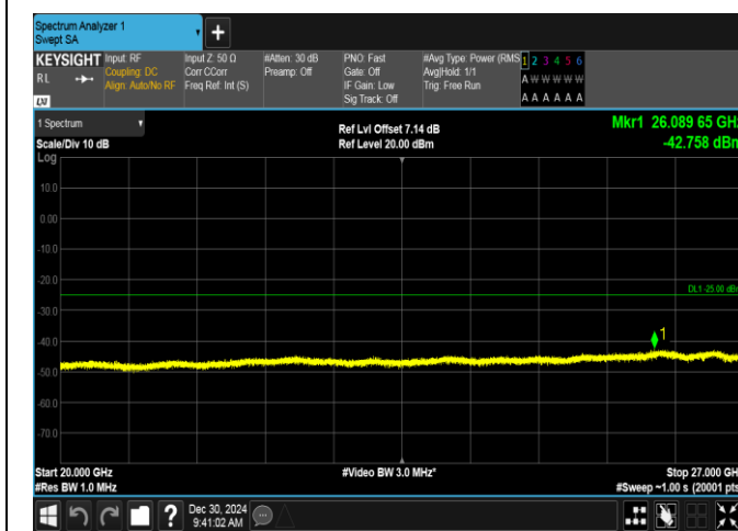
Band7-15MHz-QPSK-20825-1RB#0-20000~27000-PASS
