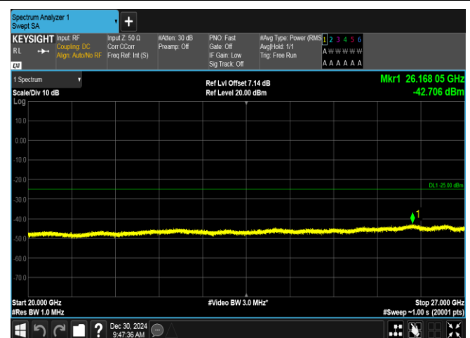
Band7-15MHz-QPSK-21100-1RB#0-20000~27000~PASS
