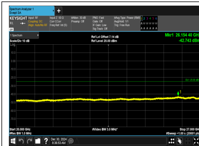
Band7-10MHz-QPSK-20800-50RB#0-20000~27000-PASS
