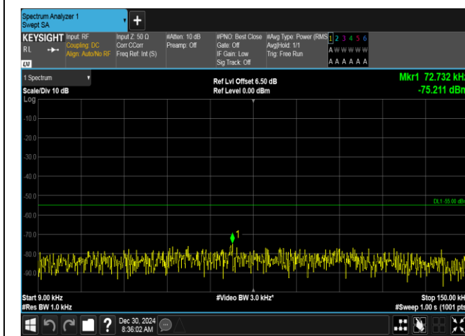
Band7-10MHz-QPSK-20800-50RB#0-0.009~0.15-PASS
