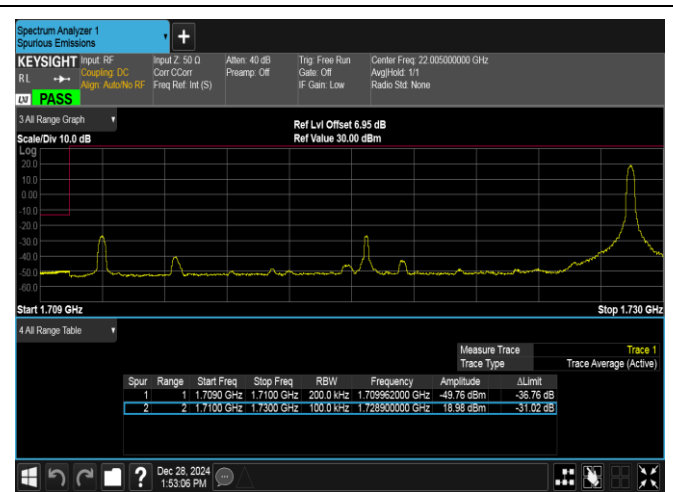
Band4-20MHz-QPSK-20050-1RB#99-PASS
