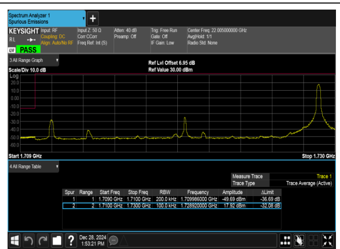
Band4-20MHz-16QAM-20050-1RB#99-PASS
