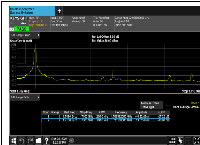
Band4-20MHz-QPSK-20050-1RB#0-PASS
