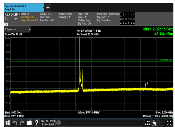
Band2-20MHz-QPSK-18700-1RB#0-1000~3000-PASS
