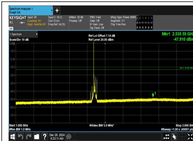
Band2-20MHz-QPSK-18900-1RB#0-1000~3000-PASS
