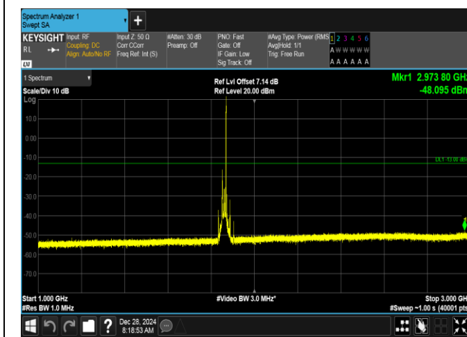
Band2-20MHz-QPSK-18700-1RB#99-1000~3000-PASS
