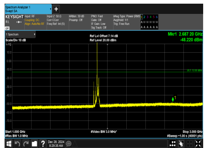
Band2-20MHz-QPSK-19100-1RB#0-1000~3000-PASS
