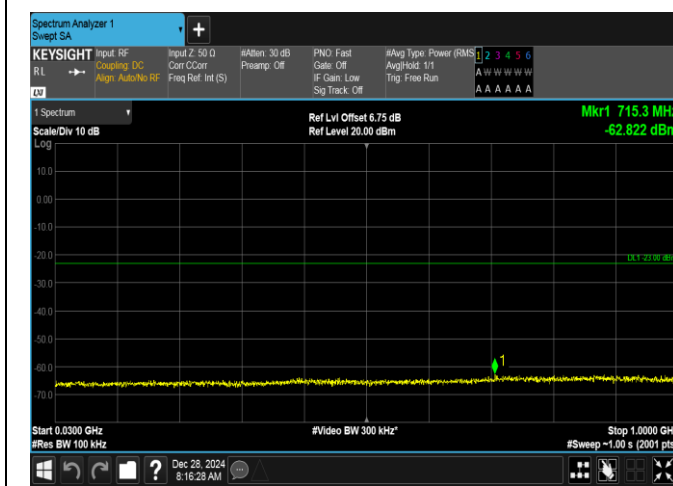
Band2-20MHz-QPSK-18700-1RB#0-30~1000-PASS
