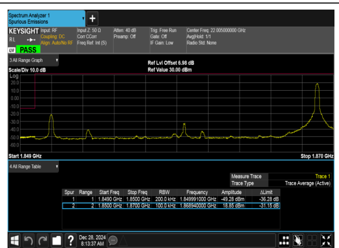
Band2-20MHz-QPSK-18700-1RB#99-PASS
