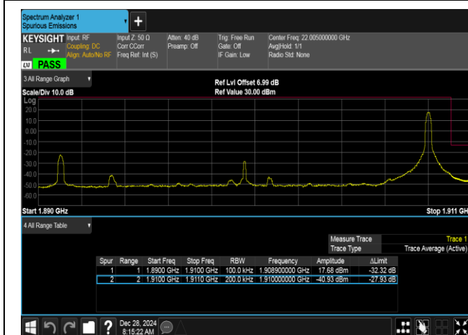
Band2-20MHz-16QAM-19100-1RB#99-PASS
