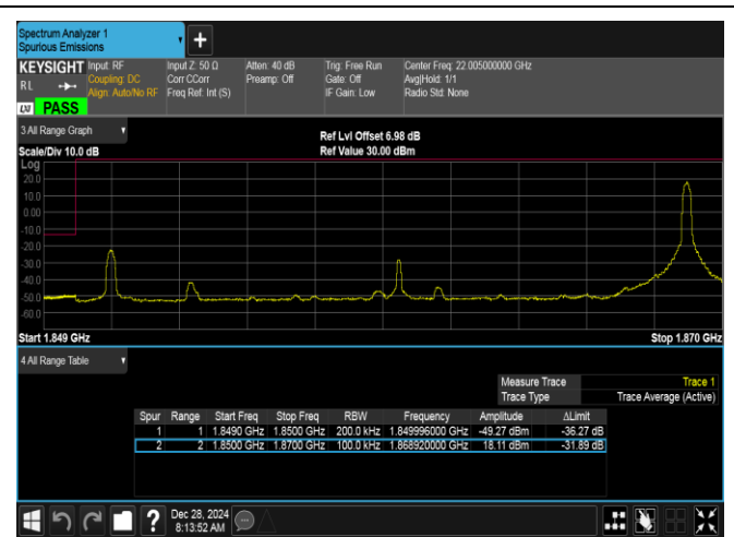
Band2-20MHz-16QAM-18700-1RB#99-PASS
