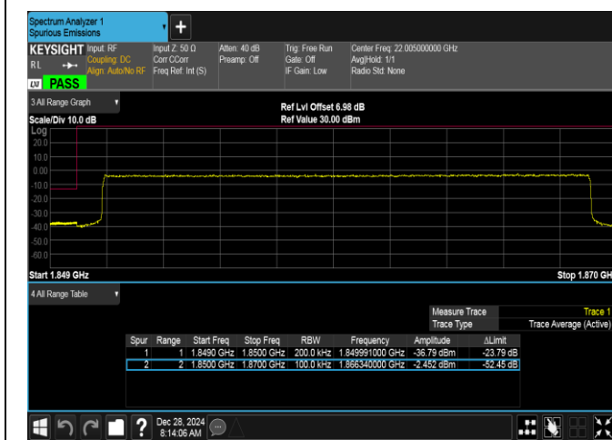
Band2-20MHz-QPSK-18700-100RB#0-PASS
