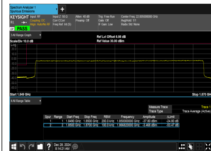
Band2-20MHz-16QAM-18700-100RB#0-PASS
