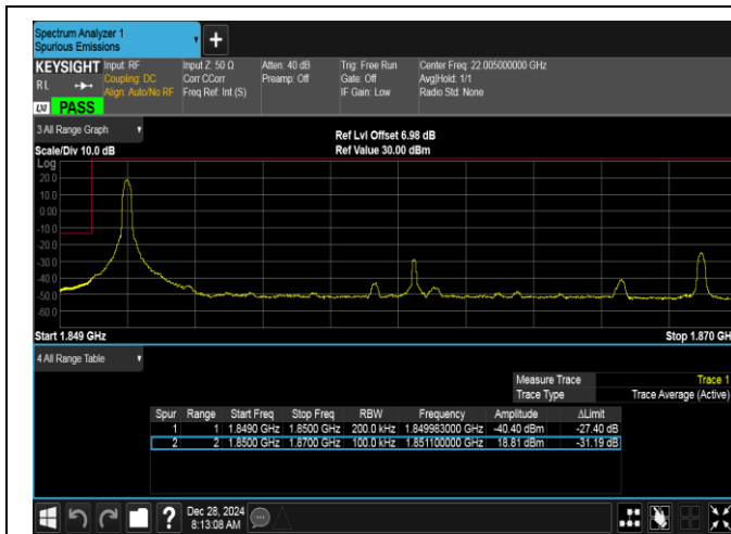
Band2-20MHz-QPSK-18700-1RB#0-PASS
