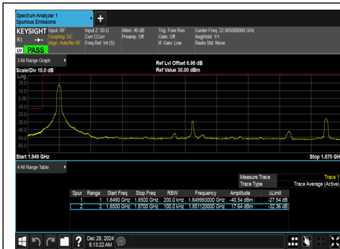
Band2-20MHz-16QAM-18700-1RB#0-PASS
