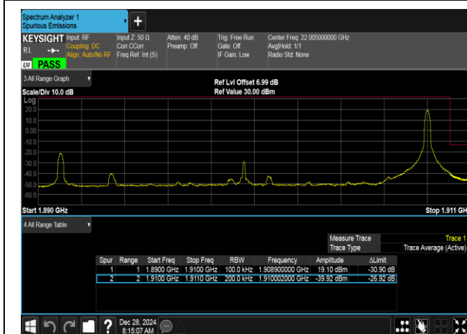
Band2-20MHz-QPSK-19100-1RB#99-PASS
