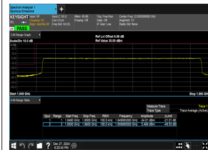
Band2-10MHz-QPSK-18650-50RB#0-PASS
