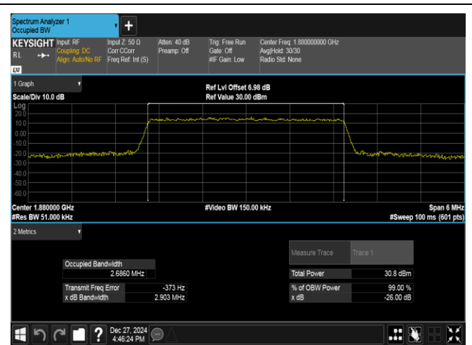
Band2-3MHz-QPSK-18900-15RB#0-PASS
