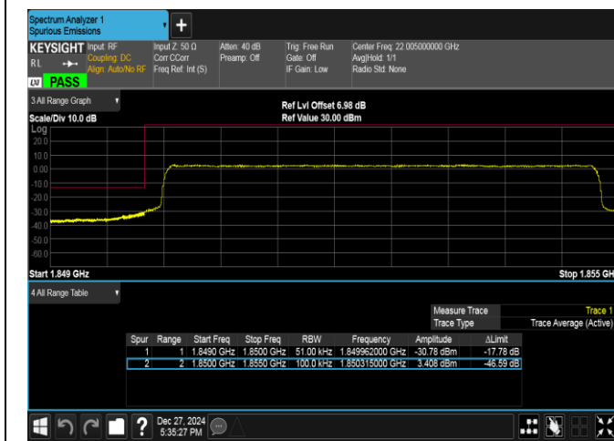
Band2-5MHz-QPSK-18625-25RB#0-PASS
