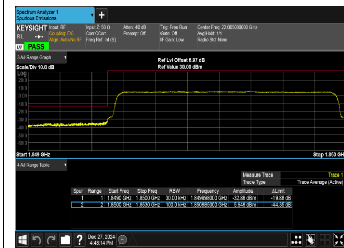
Band2-3MHz-QPSK-18615-15RB#0-PASS
