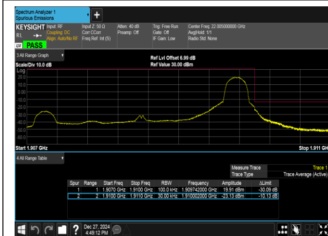
Band2-3MHz-QPSK-19185-1RB#14-PASS
