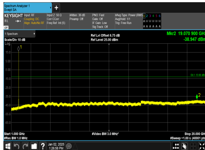
Band4-1312-5-1000~20000MHz-PASS
