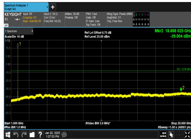
Band4-1312-1-1000~20000MHz-PASS
