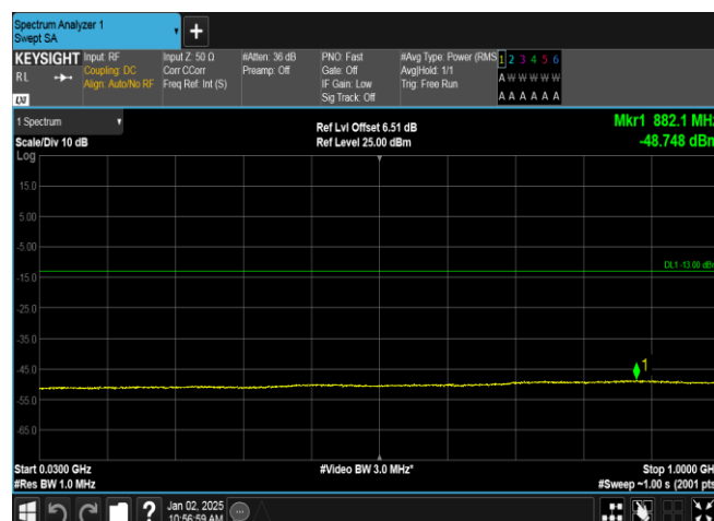
Band4-1312-4-30~1000MHz-PASS
