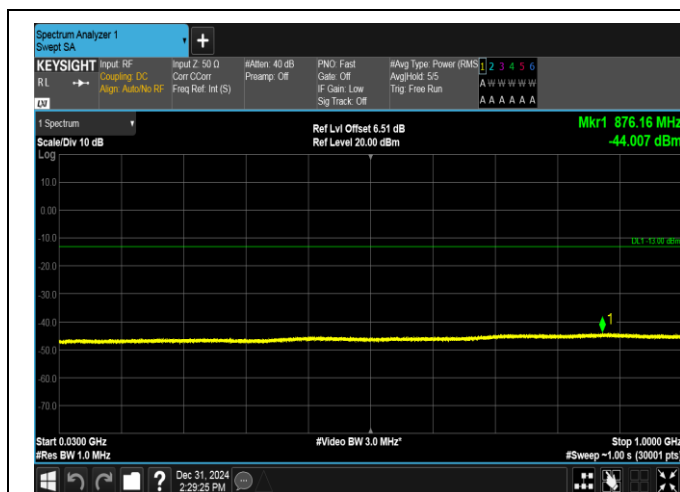
EGPRS1900-512-2-30~1000MHz-PASS
