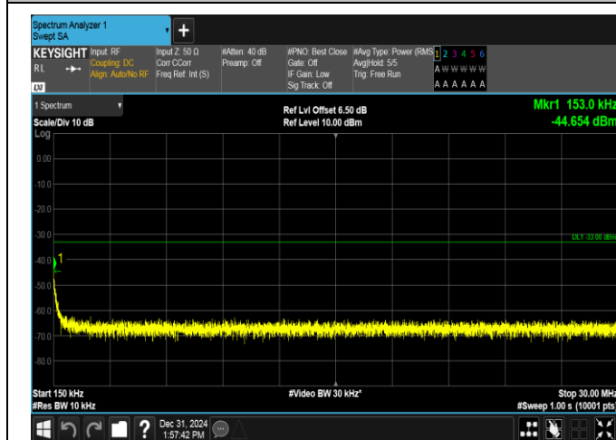
GSM1900-810-0-0.15~30MHz-PASS
