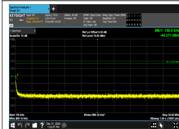
GSM850-251-5-0.15~30MHz-PASS
