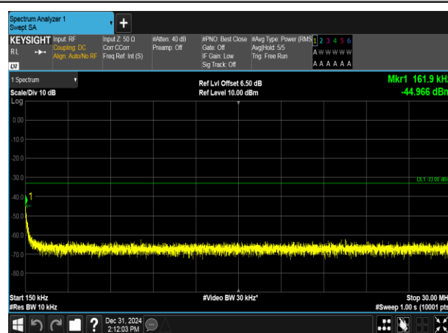
GPRS1900-512-0-0.15~30MHz-PASS
