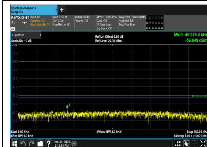
GPRS1900-661-0-0.009~0.15MHz-PASS
