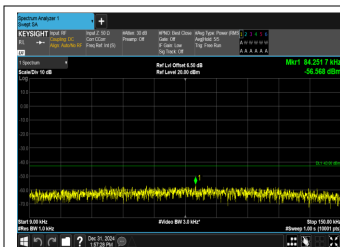
GSM1900-810-0-0.009~0.15MHz-PASS
