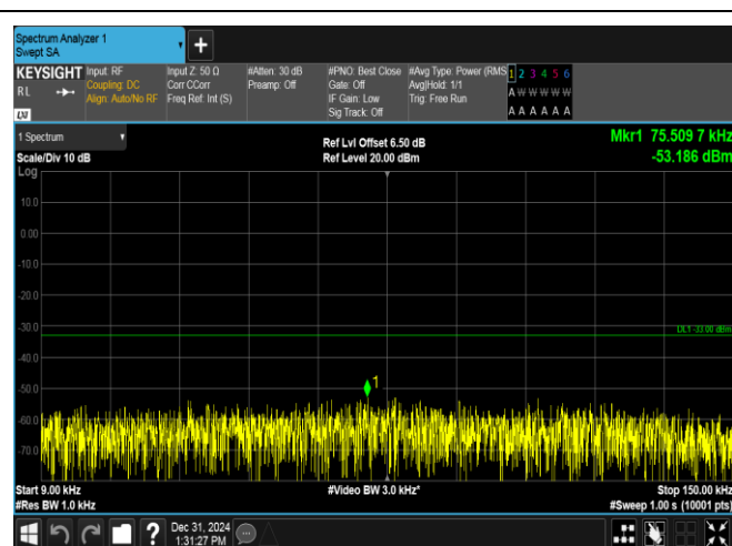
GPRS850-251-5-0.009~0.15MHz-PASS
