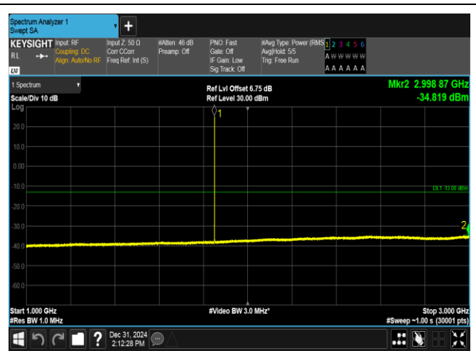
GPRS1900-512-0-1000~3000MHz-PASS
