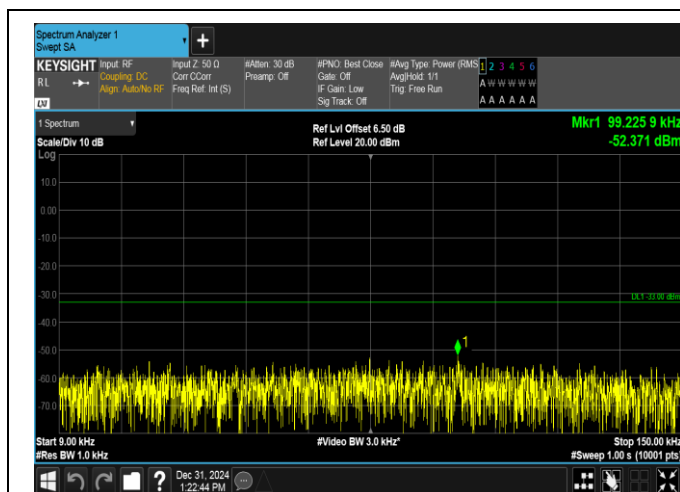
GSM850-251-5-0.009~0.15MHz-PASS
