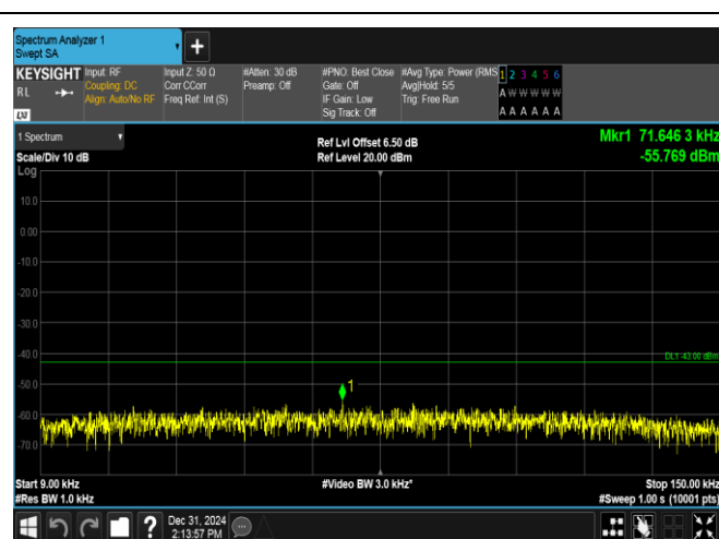
GPRS1900-810-0-0.009~0.15MHz-PASS
