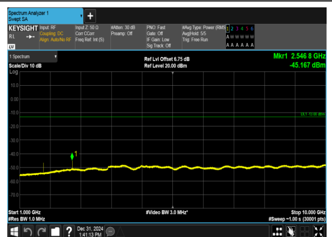
EGPRS850-251-8-1000~10000MHz-PASS
