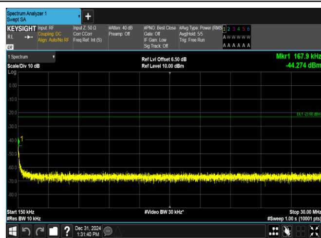
GPRS850-251-5-0.15~30MHz-PASS
