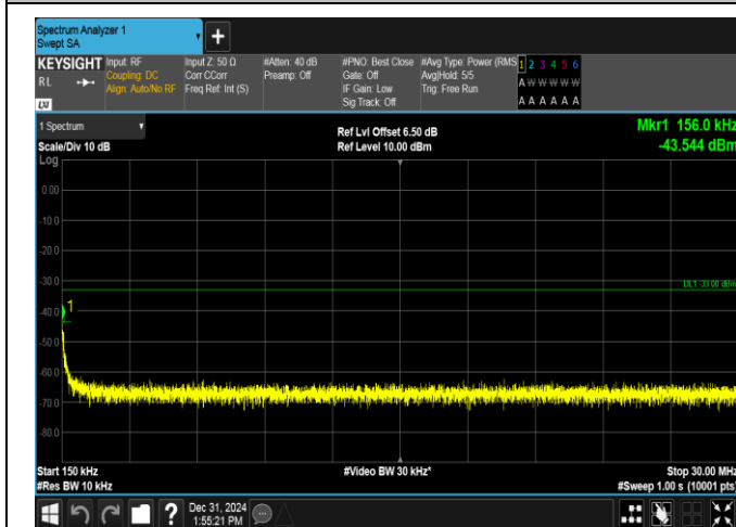
GSM1900-512-0-0.15~30MHz-PASS
