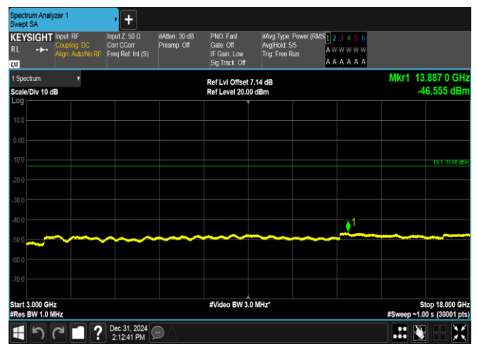
GPRS1900-512-0-3000~18000MHz-PASS
