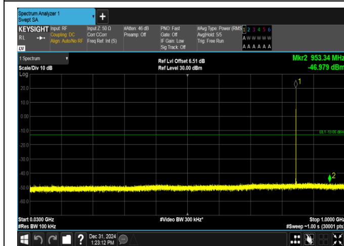
GSM850-251-5-30~1000MHz-PASS
