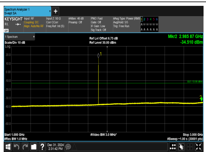
EGPRS1900-810-2-1000~3000MHz-PASS
