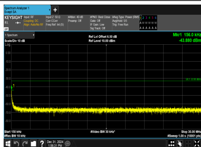
GSM1900-661-0-0.15~30MHz-PASS
