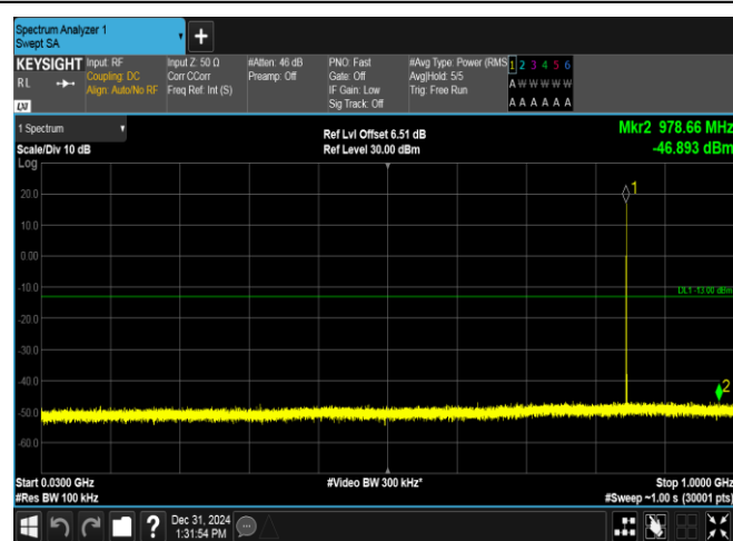
GPRS850-251-5-30~1000MHz-PASS
