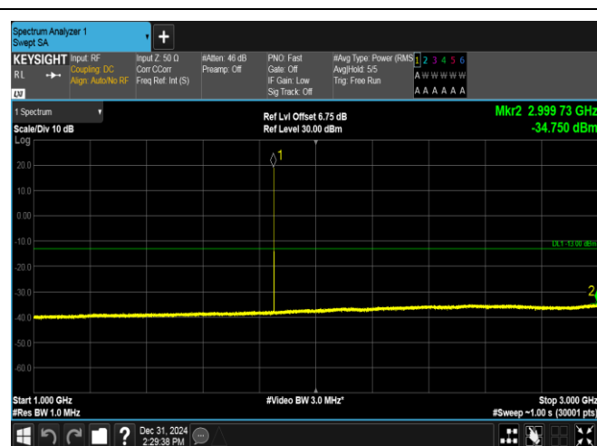
EGPRS1900-512-2-1000~3000MHz-PASS
