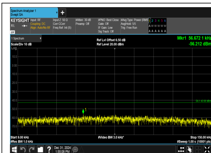
GSM1900-512-0-0.009~0.15MHz-PASS
