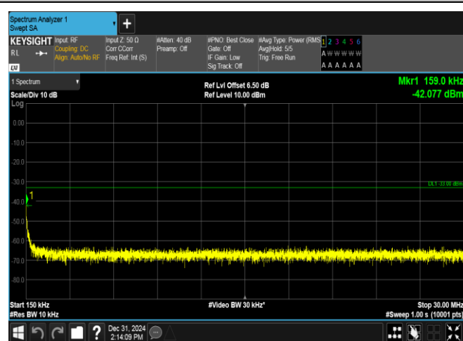
GPRS1900-810-0-0.15~30MHz-PASS
