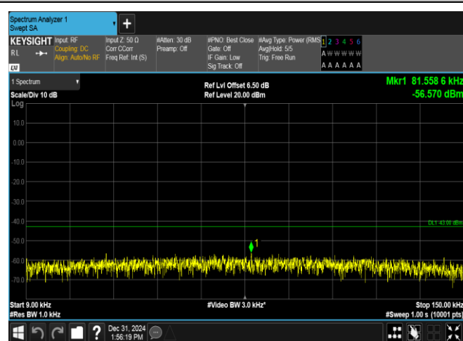
GSM1900-661-0-0.009~0.15MHz-PASS
