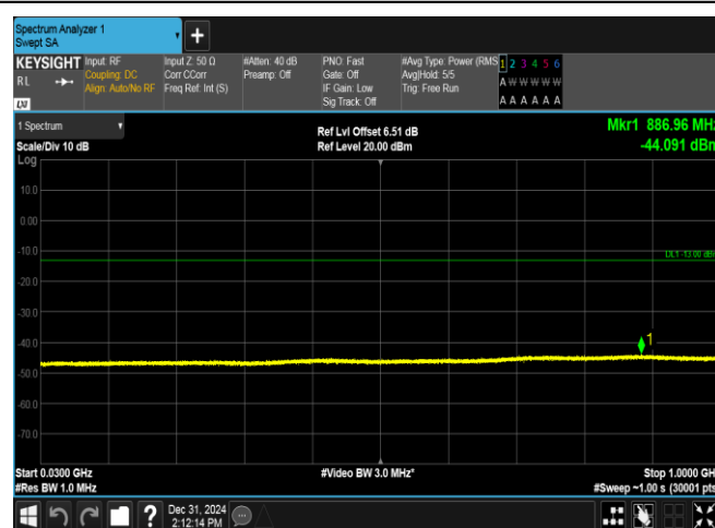
GPRS1900-512-0-30~1000MHz-PASS
