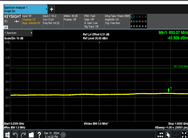
GPRS1900-810-0-30~1000MHz-PASS
