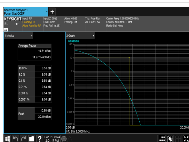
GPRS1900-661-0-PASS
