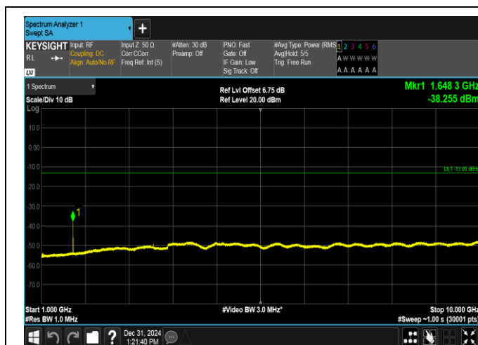
GSM850-128-5-1000~10000MHz-PASS
