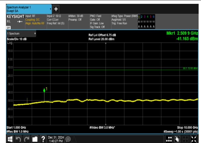
EGPRS850-190-8-1000~10000MHz-PASS
