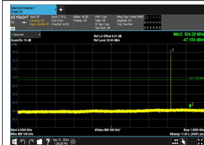
EGPRS850-128-8-30~1000MHz-PASS
