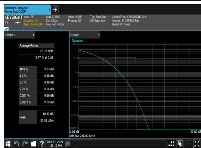
GSM1900-512-0-PASS
