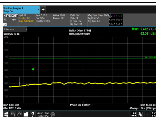
GPRS850-128-5-1000~10000MHz-PASS
