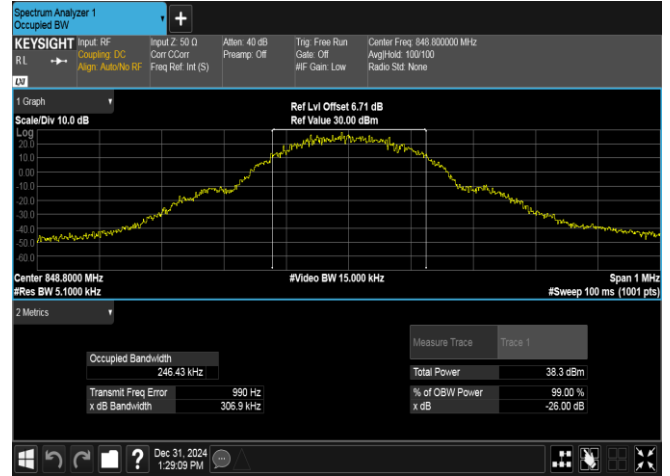
GPRS850-251-5-PASS
