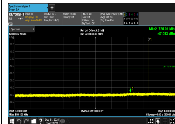
GSM850-190-5-30~1000MHz-PASS
