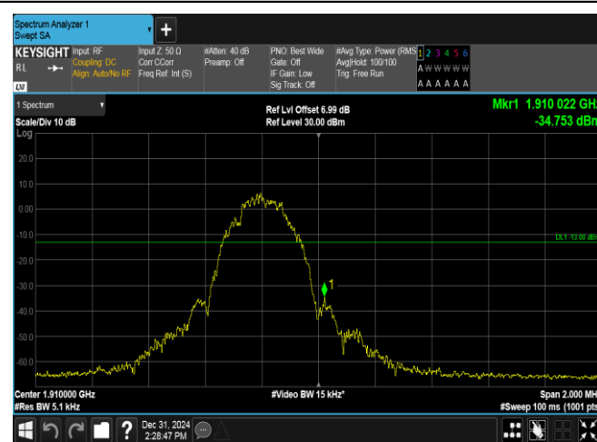
EGPRS1900-810-2-PASS
