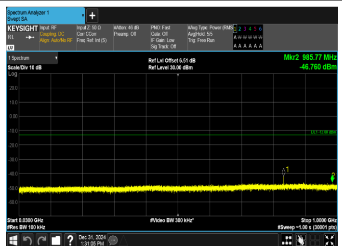
GPRS850-190-5-30~1000MHz-PASS
