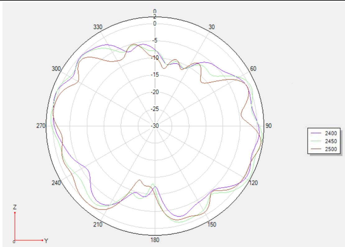
5.E 3 direction diagram/E2 面方向图
