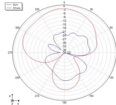
Theta=90 freq=2460MHz
