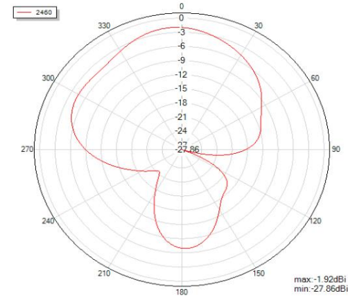
Theta=90 freq=2460MHz
