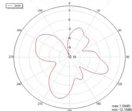
Theta=90 freq=2428MHz
