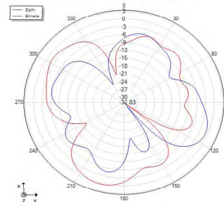
Theta=90 freq=2428MHz
