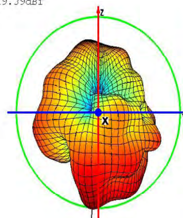
Theta=90 freq=2428MHz
